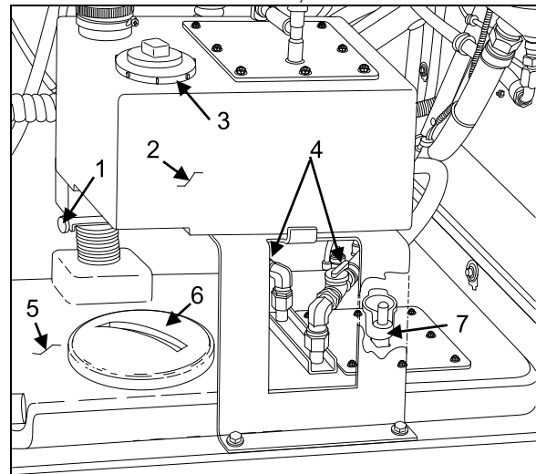
RÉSERVOIRS D'EAUX
