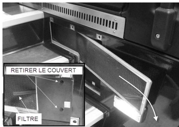
RETRAIT DU FILTRE SECTION CONDUCTEUR
