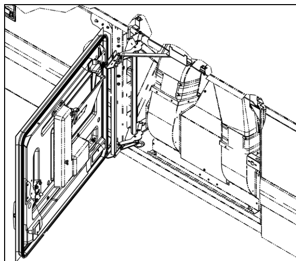
ACCÈS AU COMPARTIMENT DE L'ÉVAPORATEUR
