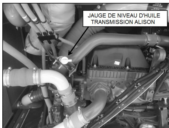
CÔTÉ GAUCHE DU MOTEUR
