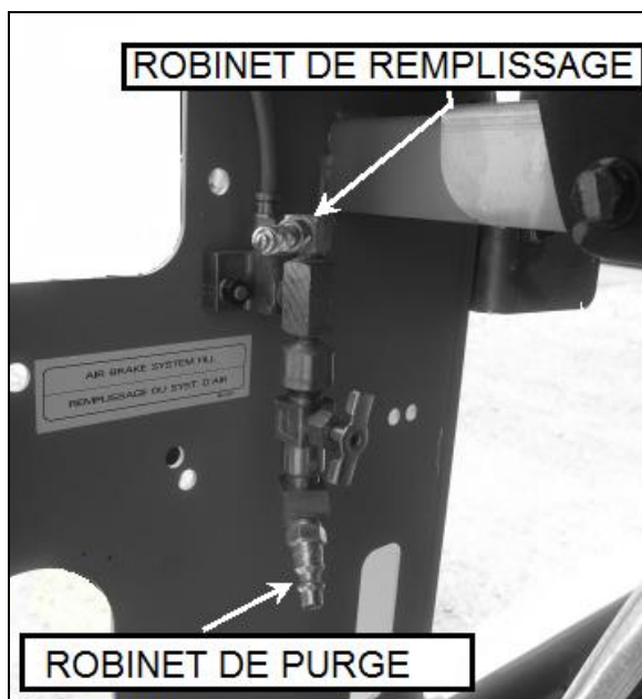
CÔTÉ DROIT DU COMPARTIMENT MOTEUR
