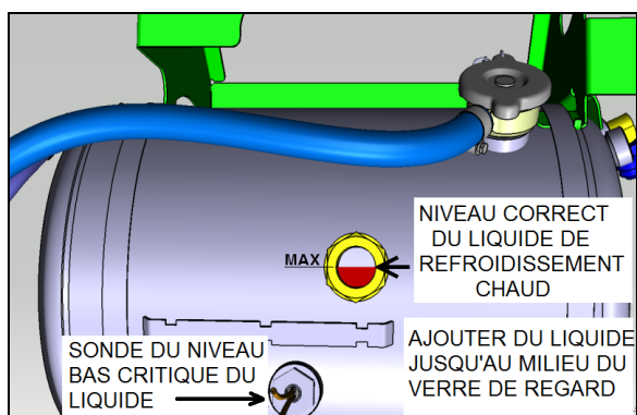
VERRE DE REGARD DU RÉSERVOIR D'EXPANSION 05094_2
