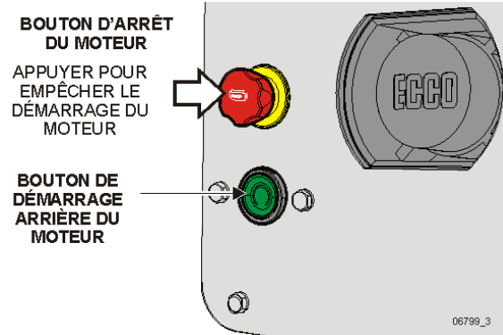
PANNEAU DE DÉMARRAGE ARRIÈRE
