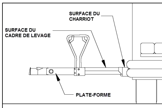
LEVAGE DU CADRE ET DU CHARRIOT À LA MÊME HAUTEUR
