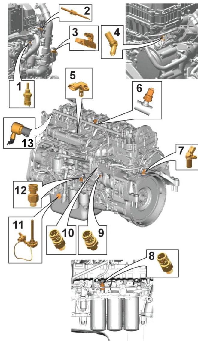
FIGURE 1 : CAPTEURS DU MOTEUR
