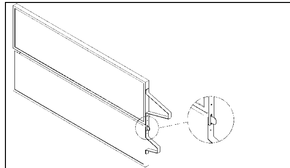
FIGURE 21 : FILTRE À AIR EN DEUX PARTIES DE L'UNITÉ DES PASSAGERS SÉRIE H:
