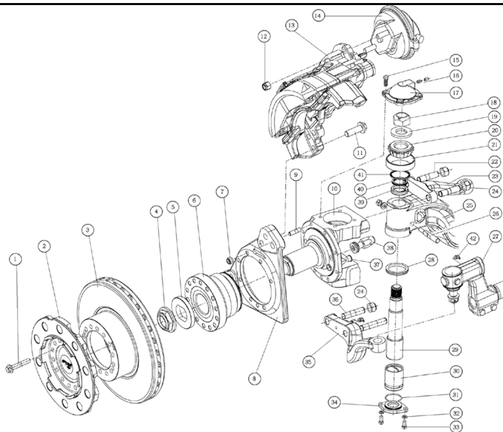
ESSIEU TYPE S84U
