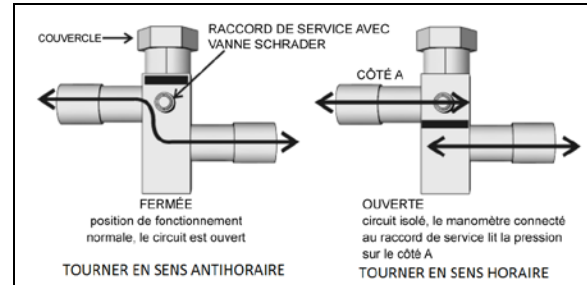
FIGURE 51 : ROBINET D'ARRÊT DU CIRCUIT DE REFROIDISSEMENT
