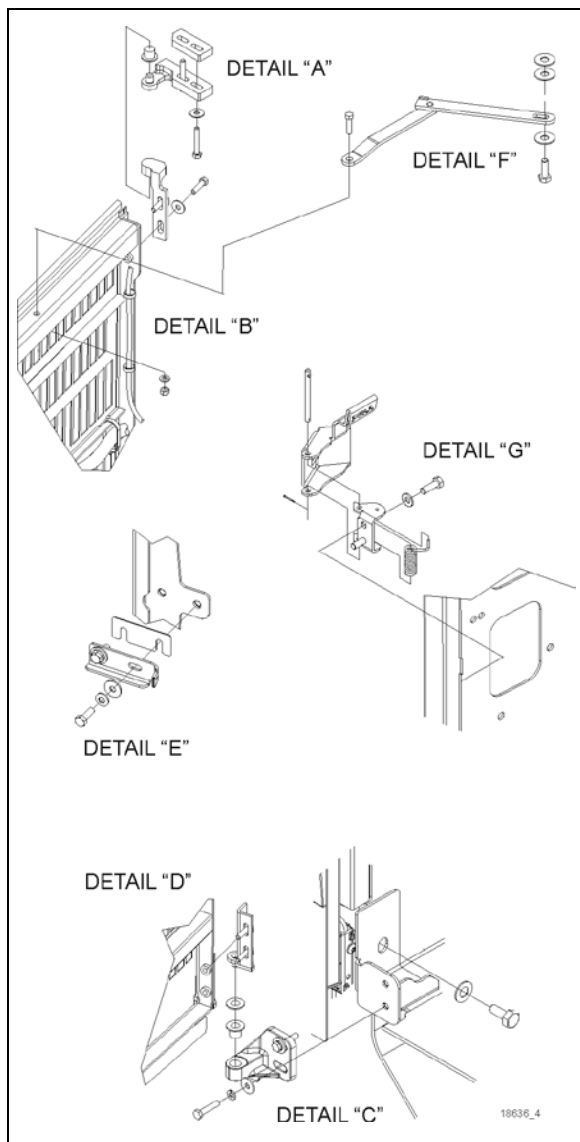
FIGURE131:PORTE DU RADIATEUR
