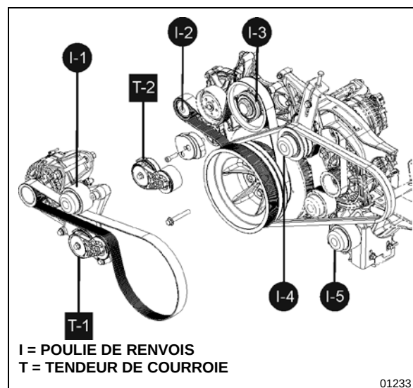
FIGURE 20 : TENDEURS DE COURROIES AUTOMATIQUES ET POULIES DE RENVOI SUR ACCESSOIRES DU MOTEUR
