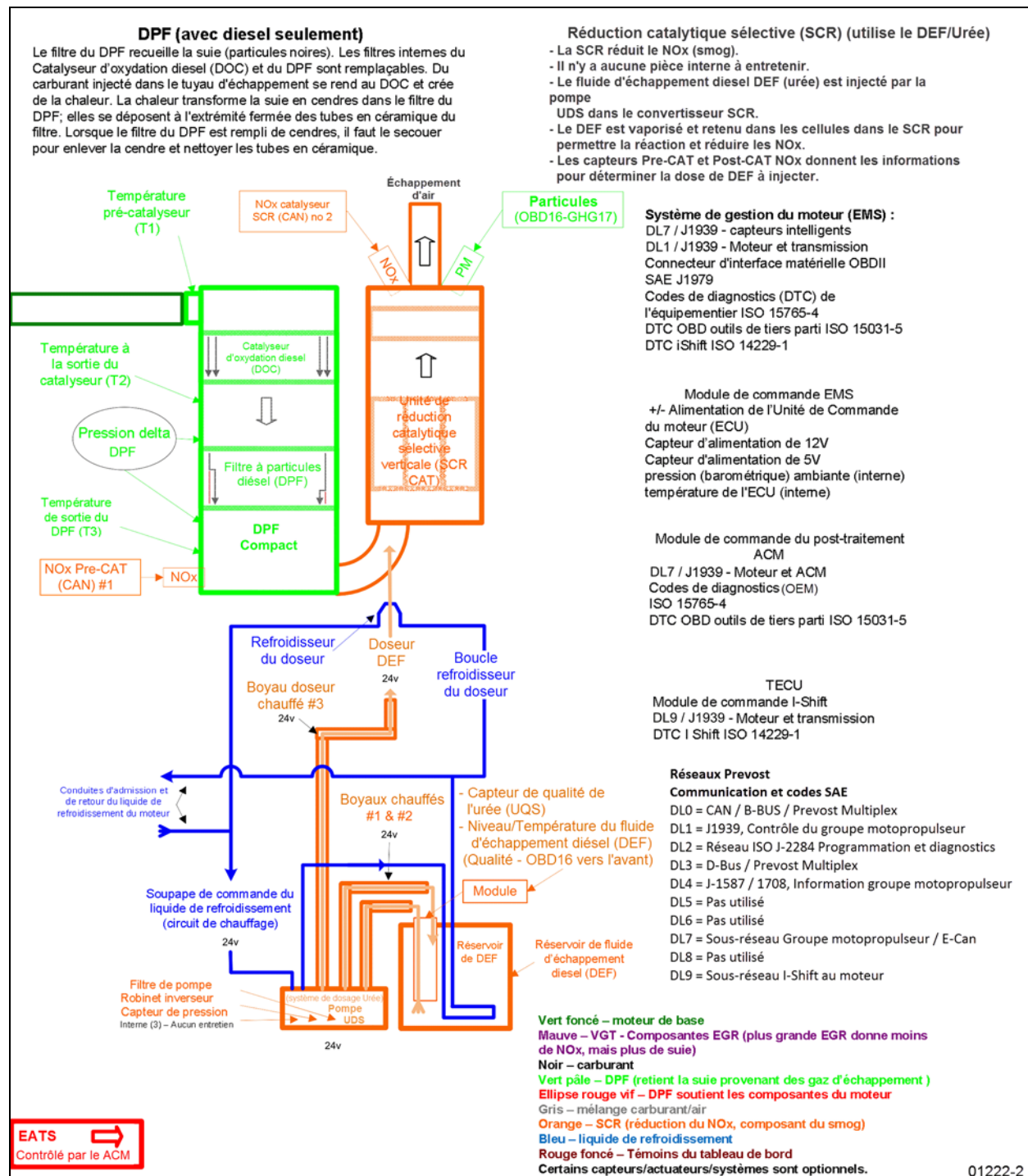
FIGURE 6 : 2010-2017 DIAGRAMME DU MOTEUR &amp; DU SYSTÈME DE POST-TRAITEMENT DES GAZ D'ÉCHAPPEMENT (2 SUR 2)
