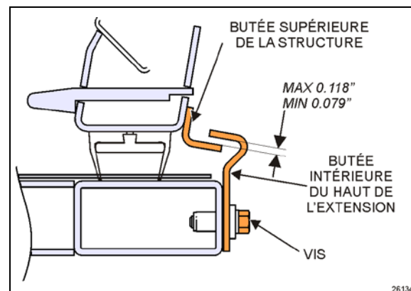
FIGURE 61: AJUSTEMENT DES BUTÉES INTÉRIEURES SUPÉRIEURES
