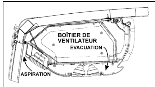
FIGURE 69 : SYSTÈME DE VENTILATION DU PORTE-BAGAGES À MAIN
