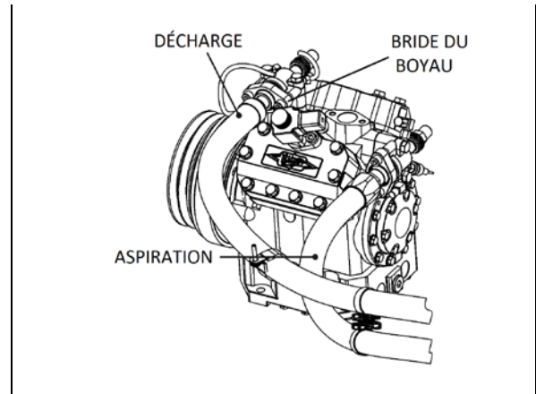
FIGURE 30: FLEXIBLE D'ASPIRATION ET DE REFOULEMENT
