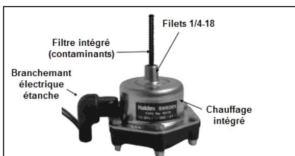
FIGURE 1: SOUPAPE DE PURGE AUTOMATIQUE
