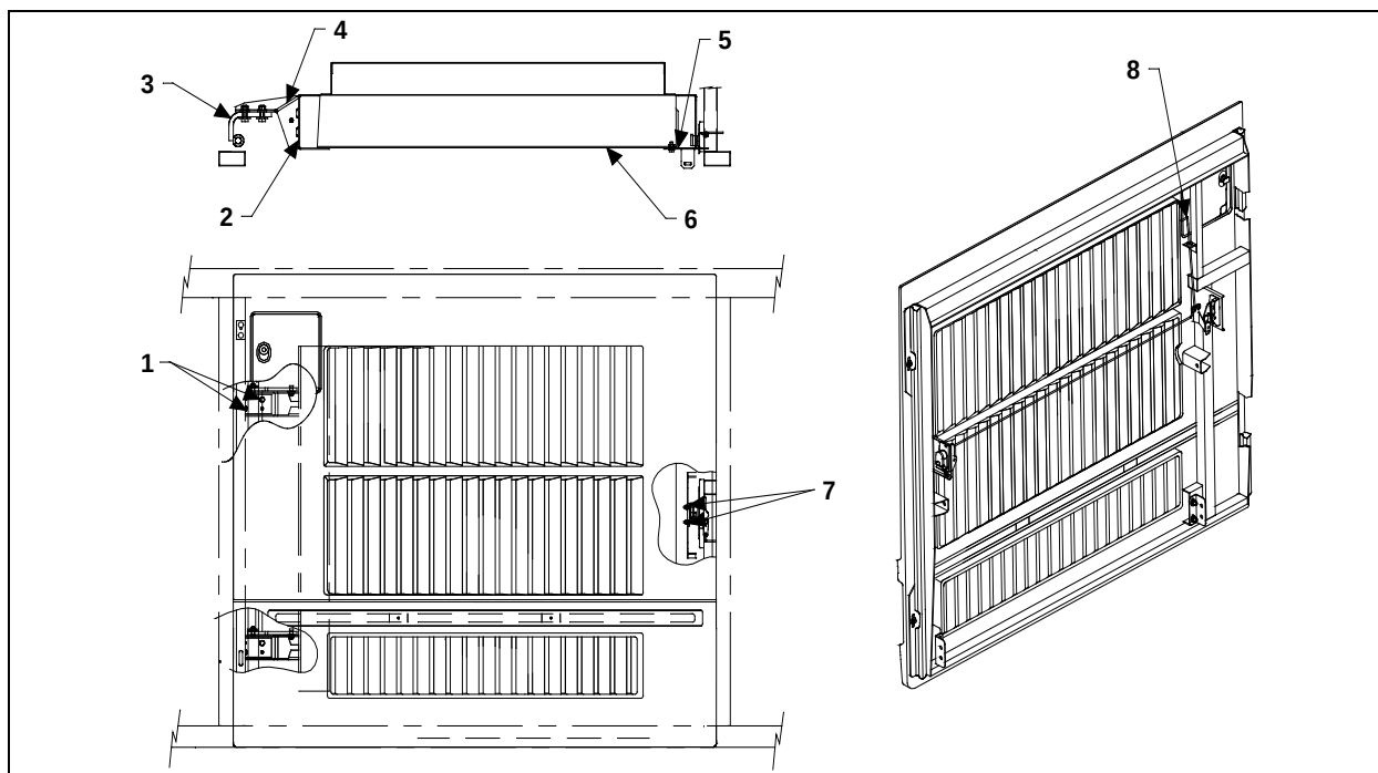
FIGURE 69 : PORTE DU COMPARTIMENT DU CONDENSEUR
