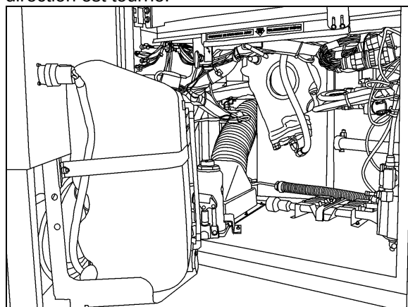
FIGURE 4 : COMPARTIMENT DE SERVICE AVANT 18611
