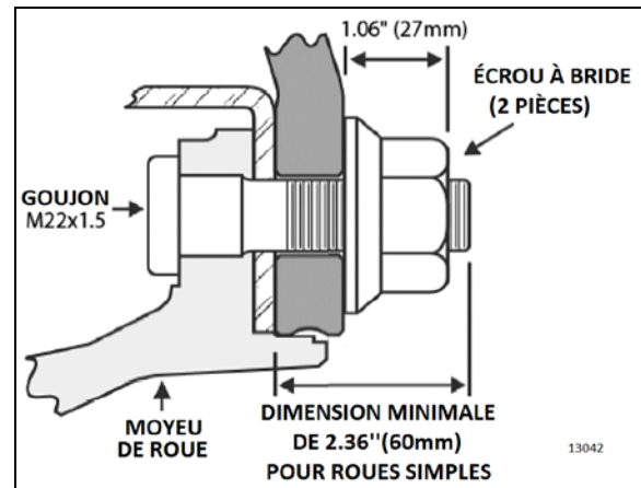
FIGURE 6 : ROUE SIMPLE
