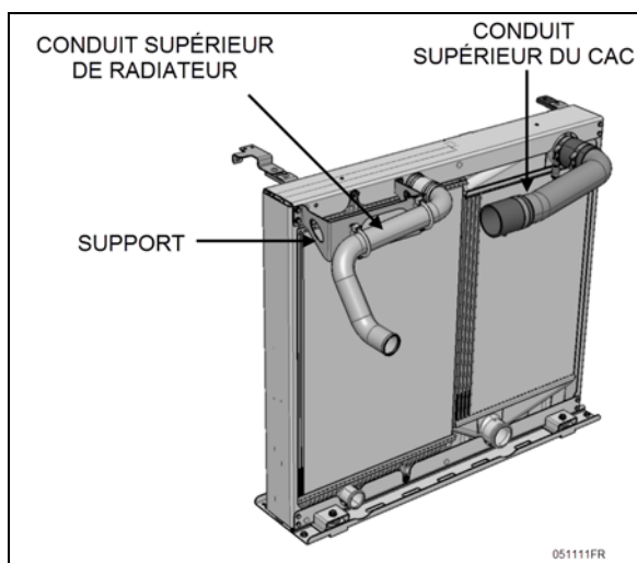
FIGURE 57: INSTALLATION DES TUYAUX, SUPPORTS ET ATTACHES DU REFROIDISSEUR D'AIR ET DU RADIATEUR
