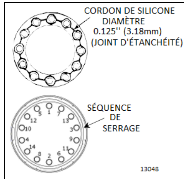
FIGURE 26 : SÉQUENCE DE SERRAGE DE bride D'ESSIEU
