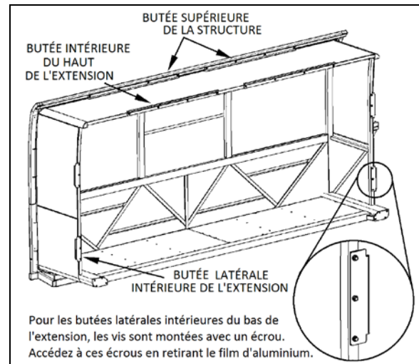
FIGURE 3: RALLONGE COULISSANTE AVANT 26059
