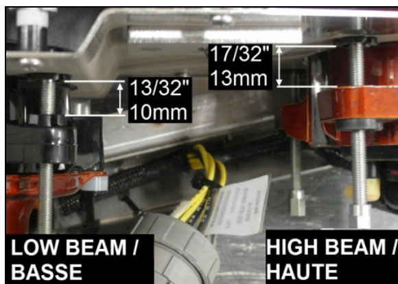
FIGURE 74: RÉGLAGE DE LA HAUTEUR DU PROJECTEUR
