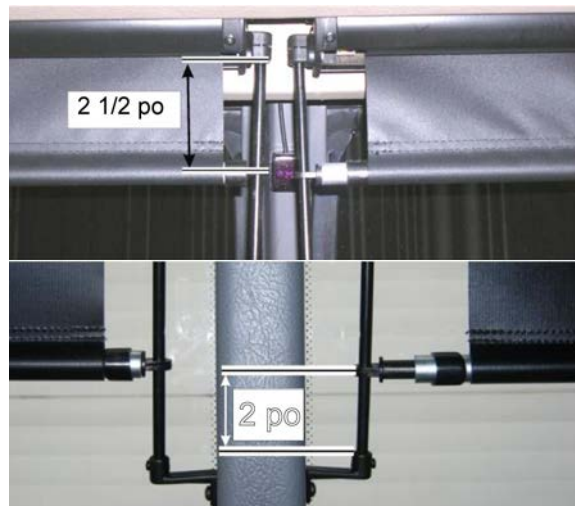
FIGURE 21: AJUSTEMENT D'USINE DES POSITIONS DE FIN DE COURSE SUPÉRIEURE ET INFÉRIEURE
