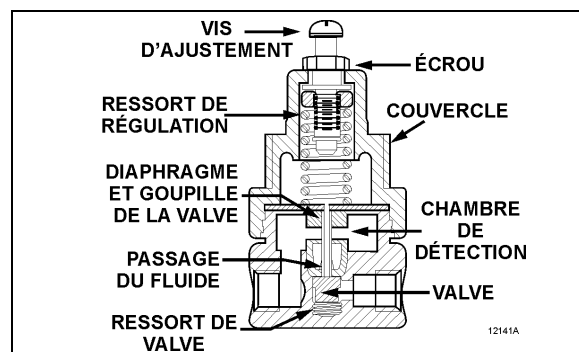
FIGURE 10: RÉGULATEUR DE PRESSION D'AIR
