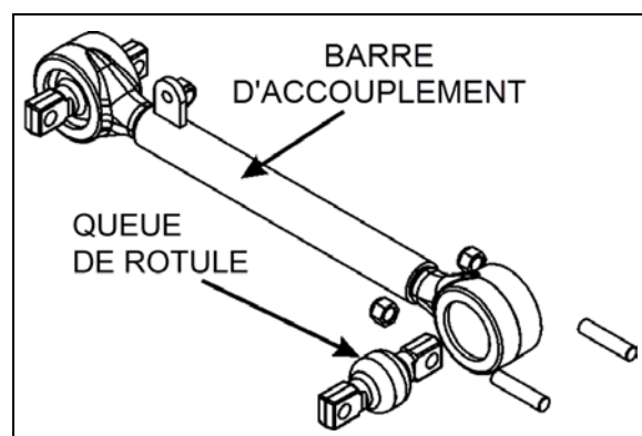
FIGURE 5: CONFIGURATION TYPE DE BARRE D'ACCOUPLEMENT
