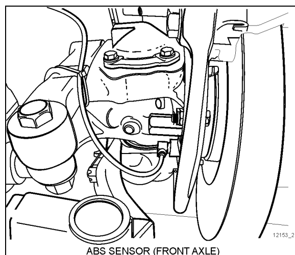
FIGURE 29: EMPLACEMENT DE CAPTEUR ABS
