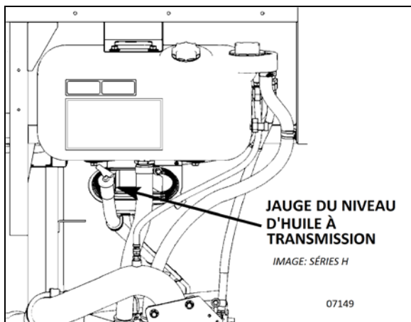
FIGURE 4: JAUGE DU NIVEAU D'HUILE (ALLISON)
