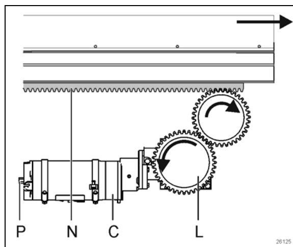
FIGURE 57 : PIGNONS DE MOTEUR D'ÉTIREMENT (AVANT ILLUSTRÉ)
