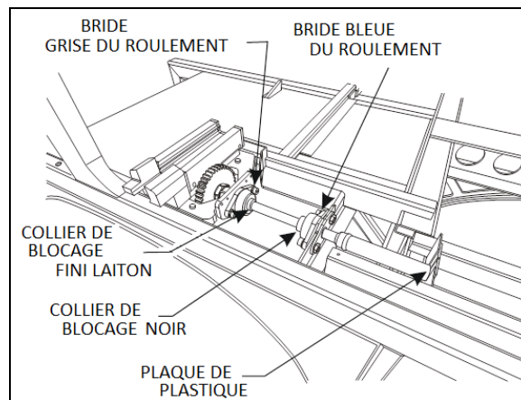
FIGURE 15: ORGANES MÉCANIQUES (TYPES) 26154
