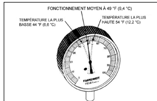
FIGURE 58: OSCILLATION DE TEMPÉRATURE HAUTE ET BASSE AU BULBE DISTANT
