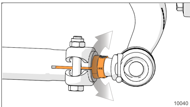
FIGURE 8: BAGUE D'AJUSTEMENT FIN
