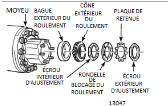
FIGURE 25 : MOYEU DE ROUE D'ESSIEU MOTEUR
