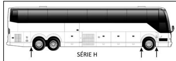
FIGURE 5: POINTS DE LEVAGE SOUS LE CHÂSSIS 18524
