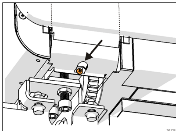
FIGURE 65: COUVERCLE FLEXIBLE DU RAIL
