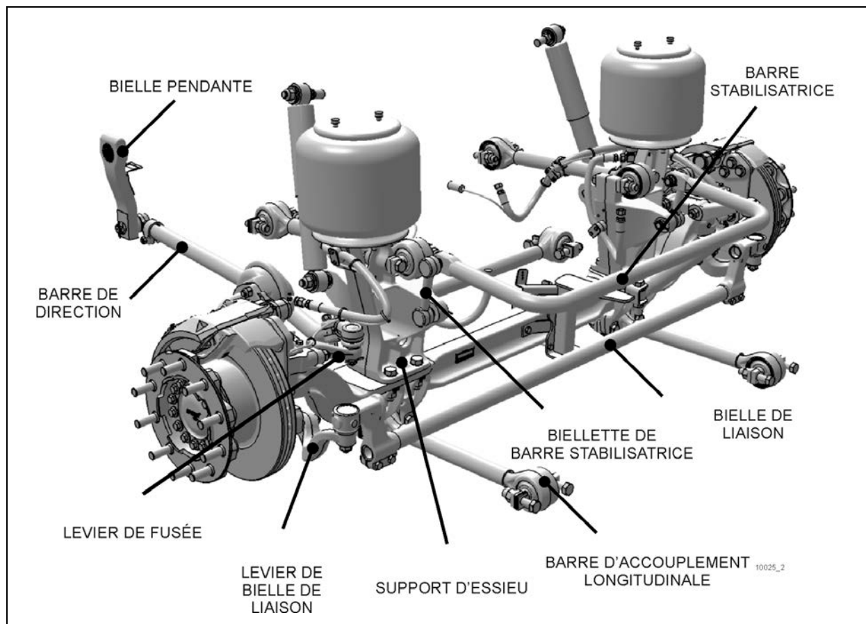
FIGURE 1: ASSEMBLAGE D'ESSIEU RIGIDE AVANT
