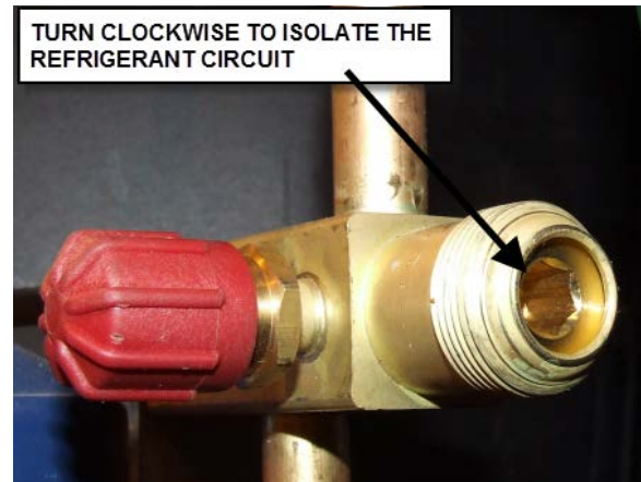
FIGURE 52 : ROBINET D'ARRÊT DU CIRCUIT DE REFROIDISSEMENT
