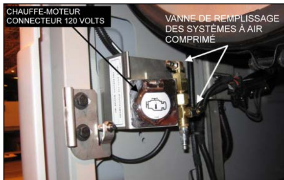
FIGURE 47: EMBLACEMENT DE SOUPAPE ARRIÈRE SUR LA SÉRIE X3
