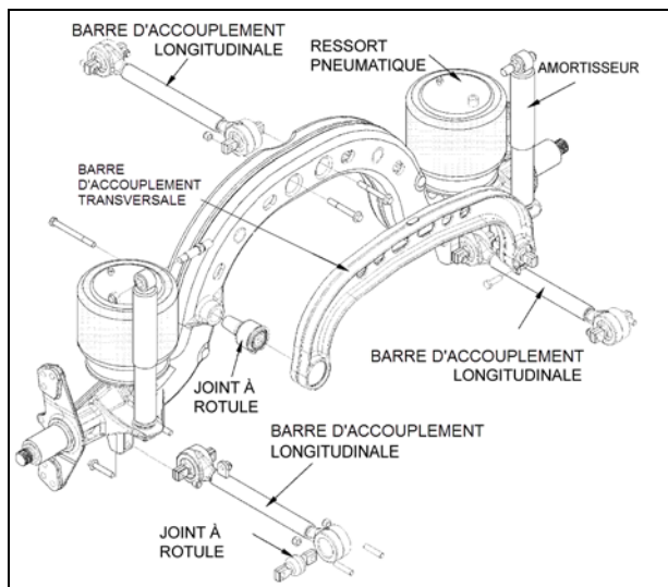
FIGURE 38 : SUSPENSION D'ESSIEU AUXILIAIRE
