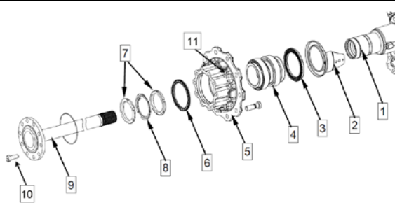
FIGURE 27: ASSEMBLAGE DE MOYEU D'ESSIEU DIRECTEUR ZF A-132
