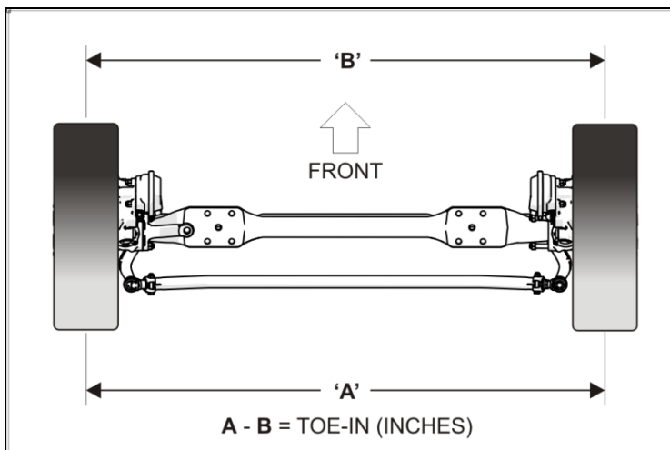
FIGURE 7: MESURE DU PINCEMENT
