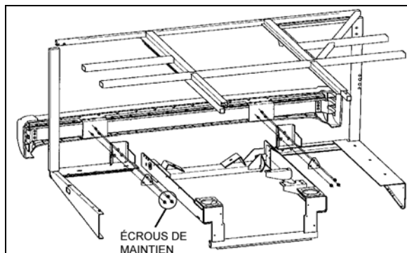
FIGURE 12: PARE-CHOCS ARRIÈRE
