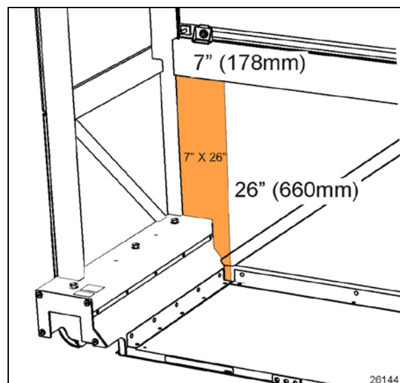
FIGURE 71: ZONE D'INTERDICTION DE PERÇAGE (AVANT ET ARRIÈRE)
