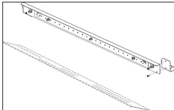
FIGURE 103: ÉCLAIRAGE D.E.L. DIRECT ET VERRE
