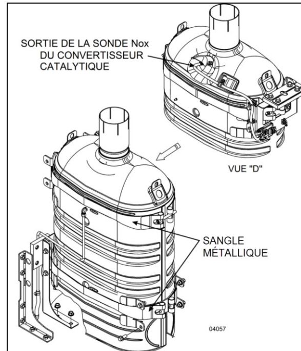
FIGURE 5: CONVERTISSEUR CATALYTIQUE
