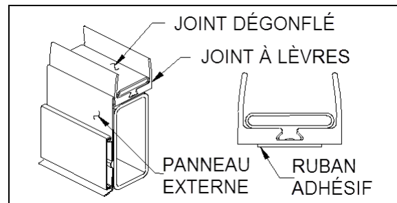
FIGURE 33: ASSEMBLAGE DU JOINT D'ÉTANCHÉITÉ 26160
