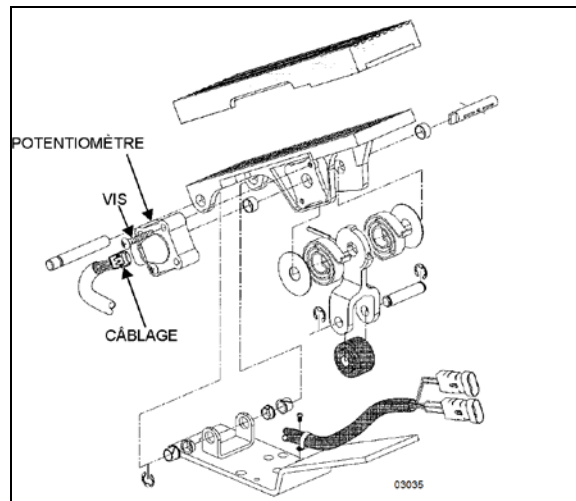
FIGURE 15 : ENSEMBLE DE PÉDALES ÉLECTRONIQUES
