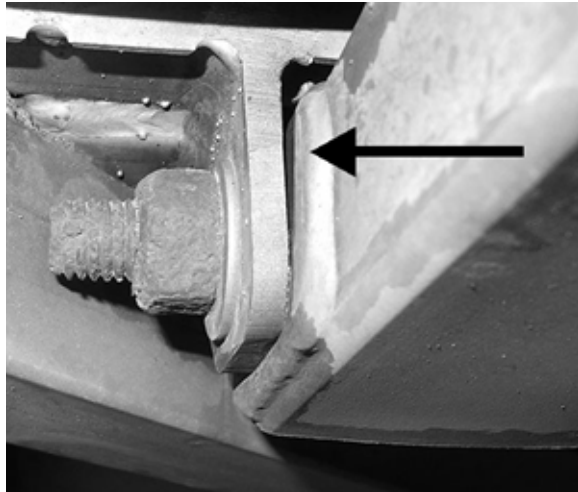
FIGURE 25: JEU VISIBLE SUR LES JOINTS TRANSVERSAUX
