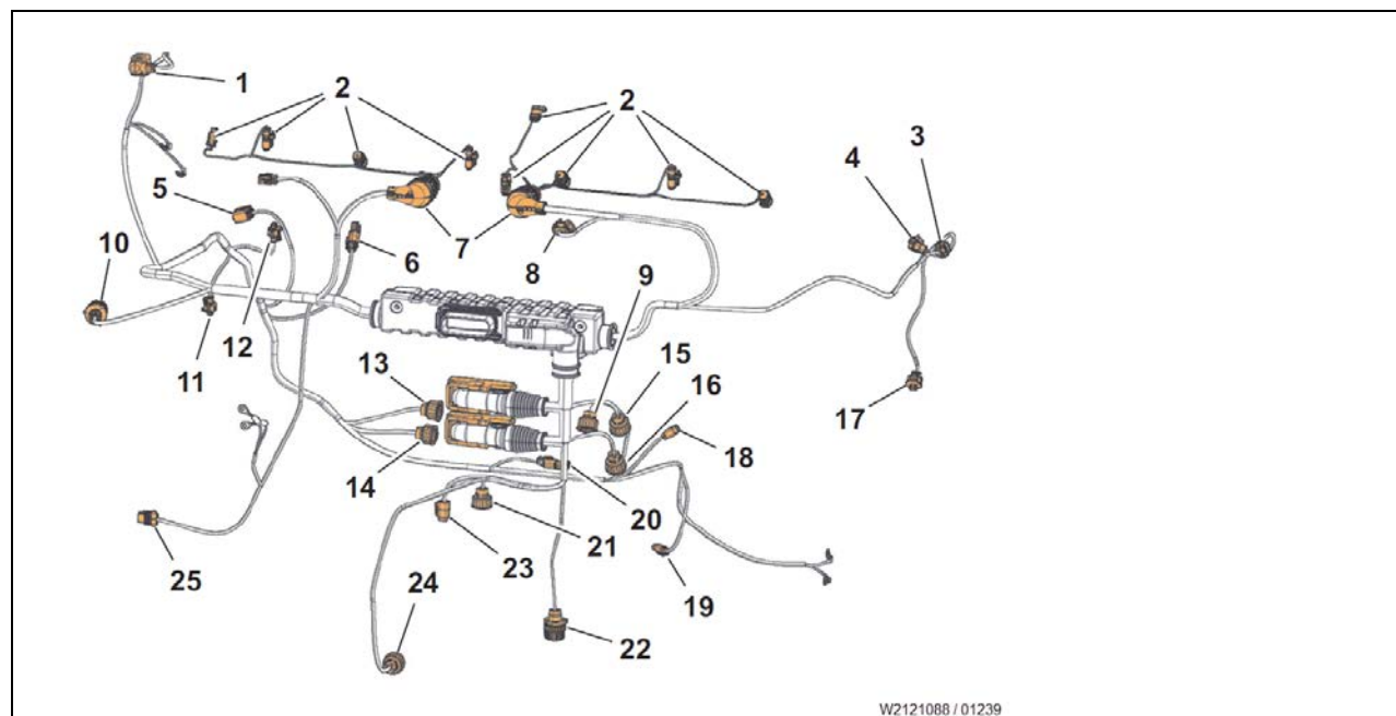
FIGURE 2 : FAISCEAU DE CÂBLES DU MOTEUR D13H
