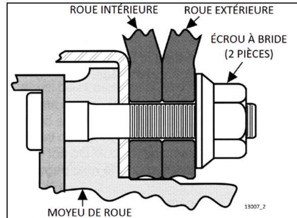
FIGURE 5 : ROUES D'ESSIEU MOTEUR
