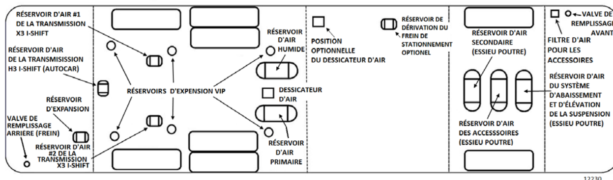
FIGURE 3: EMLACEMENTS DES RÉSERVOIRS D'AIR DE SUSPENSION RIGIDE (AVEC RÉSERVOIRS D'EXPANSION VIP)
