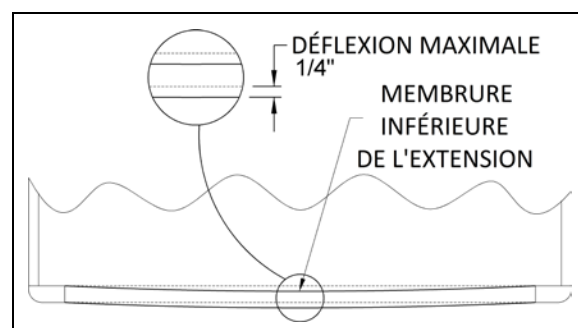
FIGURE 44: DÉFLEXION D'EXTENSION AVANT 26162
