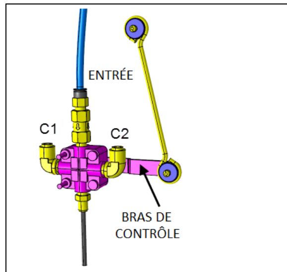
FIGURE 43 : SOUPE DE COMMANDE DE HAUTEUR
