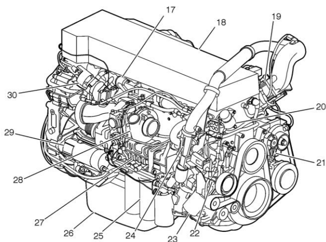
FIGURE 1 : VUE D'ENSEMBLE DU MOTEUR D13H, CÔTÉ TURBOCOMPRESSEUR
