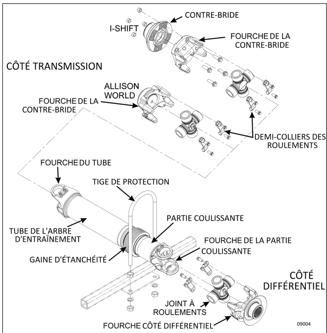
FIGURE 4 : ASSEMBLAGE DE L'ARBRE DE TRANSMISSION (TYPE)
