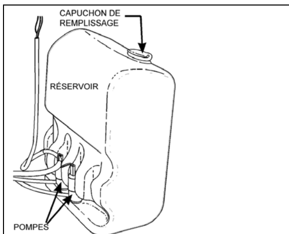
FIGURE 35: RÉSERVOIR DU LIQUIDE DE LAVE-GLACE 23220
