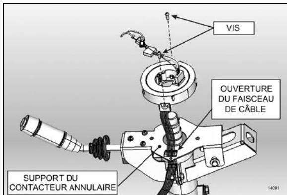
FIGURE 14 : POSE DU CONTACTEUR ANNULAIRE
