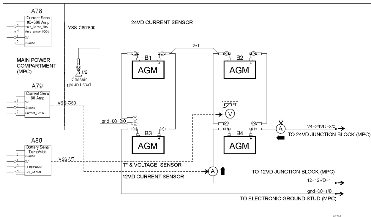
FIGURE 36: DIAGRAMME DES CONNEXIONS DES BATTERIES – SÉRIE X3
