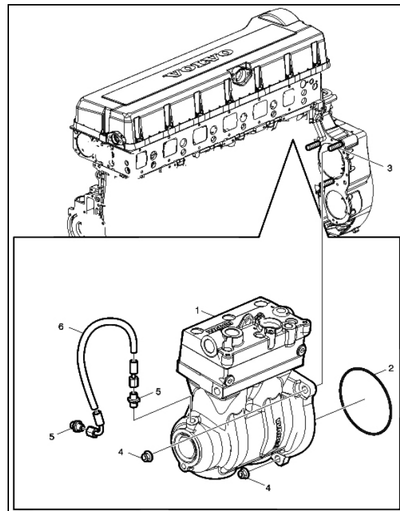
FIGURE 12 : EMBLACEMENT DU COMPRESSEUR D'AIR
