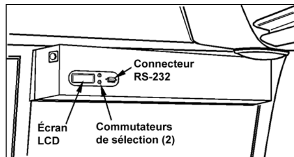
FIGURE 18: RIDEAU DE DESTINATION ÉLECTRONIQUE 23123
