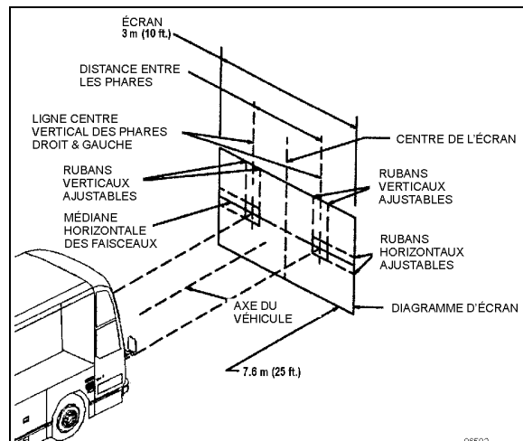
FIGURE 81 : ALIGNEMENT DE L'ÉCRAN DE RÉGLAGE DES PHARES
