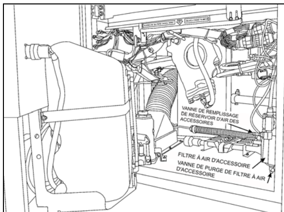
FIGURE 49: EMPLACEMENT DE LA SOUPAPE AVANT SUR LA SÉRIE X3 12210
