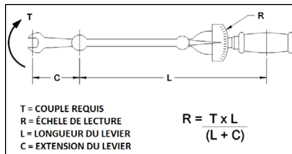
FIGURE 17: ÉQUATION POUR CLÉ DYNAMOMÉTRIQUE 26155
