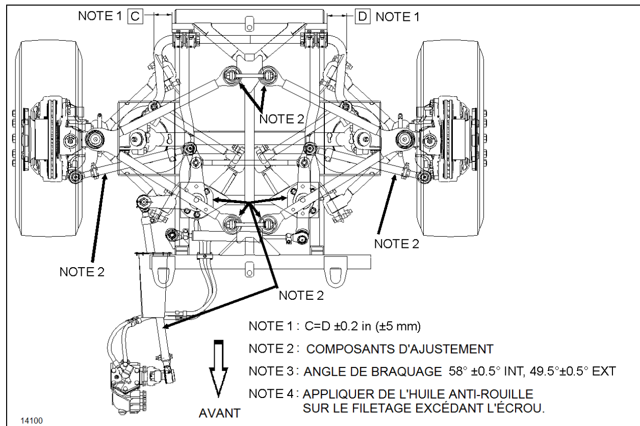
FIGURE 25: GÉOMÉTRIE IFS
