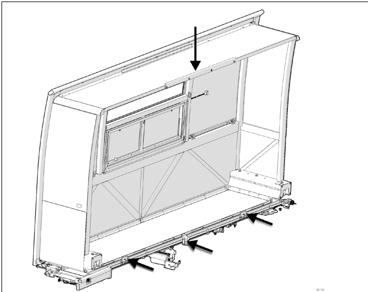
FIGURE 60: BUTÉES
