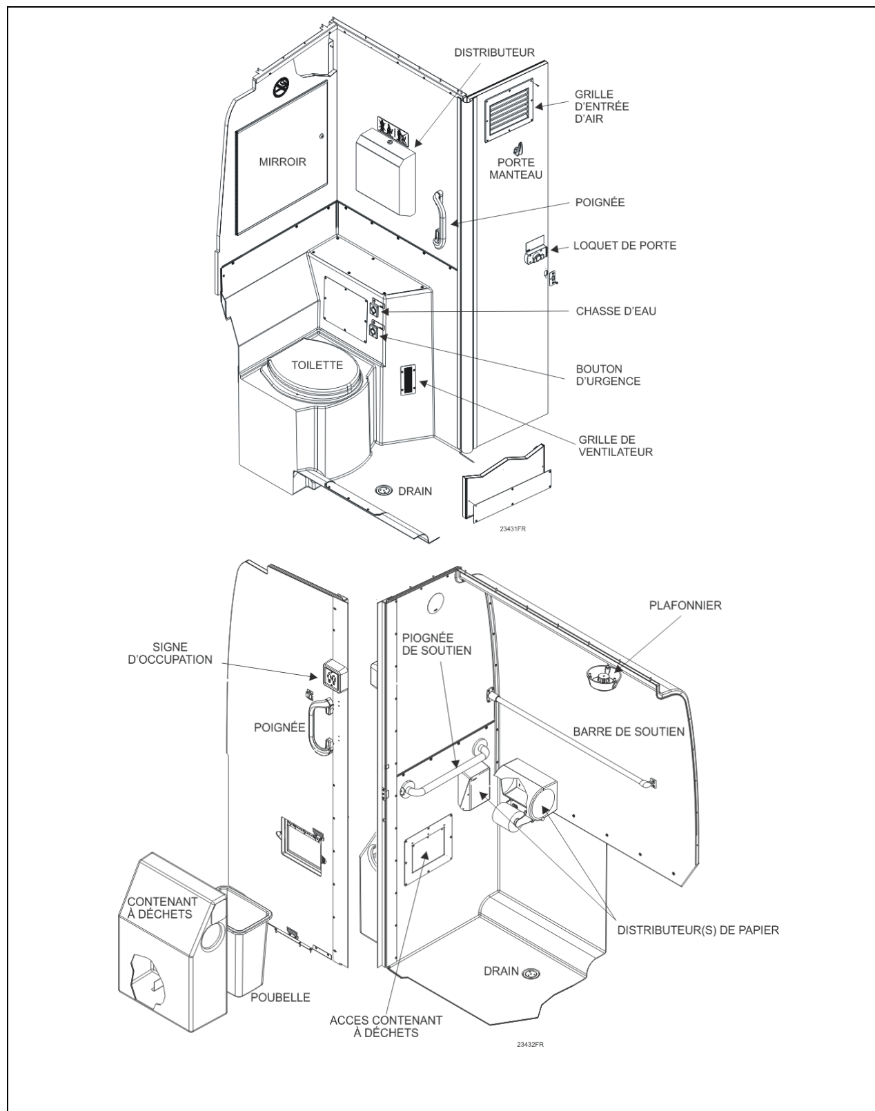
FIGURE 23 : CABINET D'AISANCES
