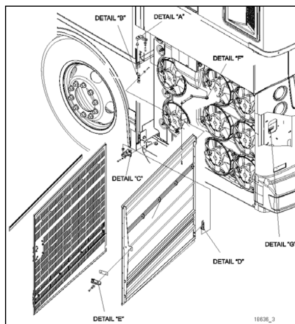
FIGURE130:PORTE DU RADIATEUR
