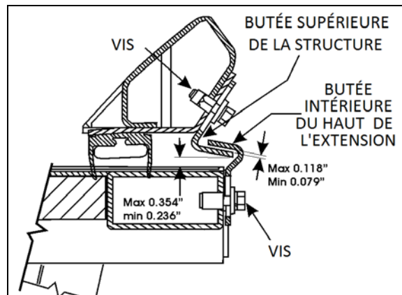
FIGURE 6: RÉGLAGE DES BUTÉES INTÉRIEURES SUPÉRIEURES 26147
