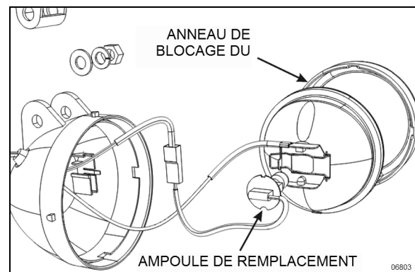
FIGURE 93 : VUE ÉCLATÉE DU PHARE ANTIBROUILLARD
