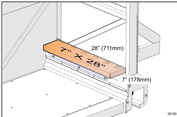
FIGURE 50: ZONE DE PERÇAGE INTERDIT, RALLONGE AVANT DROITE
