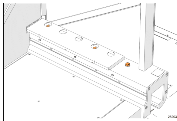
FIGURE 44: VIS SUPÉRIEURES DU RAIL
