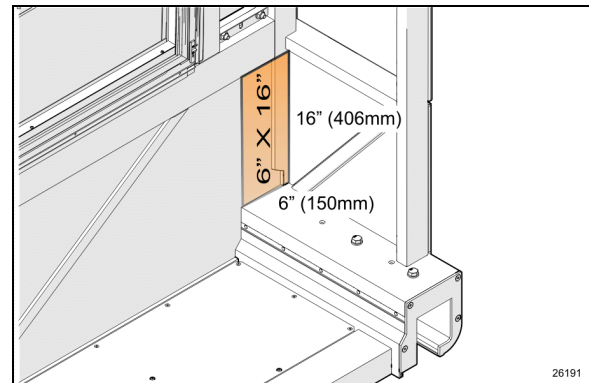
FIGURE 52: ZONE DE PERÇAGE INTERDIT, RALLONGE ARRIÈRE DROITE
