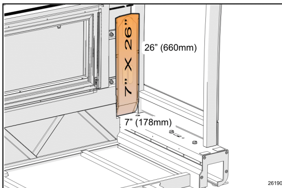
FIGURE 51: ZONE DE PERÇAGE INTERDIT, RALLONGE ARRIÈRE GAUCHE
