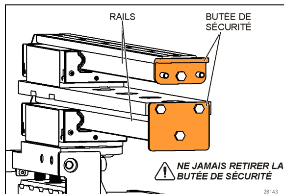
FIGURE 67: BUTÉES DE SÉCURITÉ SUR LES RAILS
