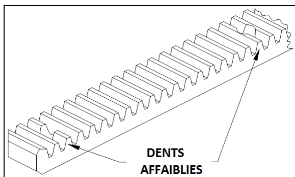
FIGURE 31: CRÉMAILLÈRE 26151
