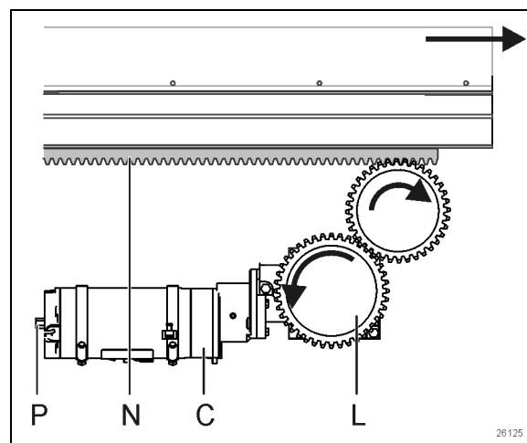
FIGURE 56 : PIGNONS DE MOTEUR D'ÉTIREMENT (AVANT ILLUSTRÉ)
