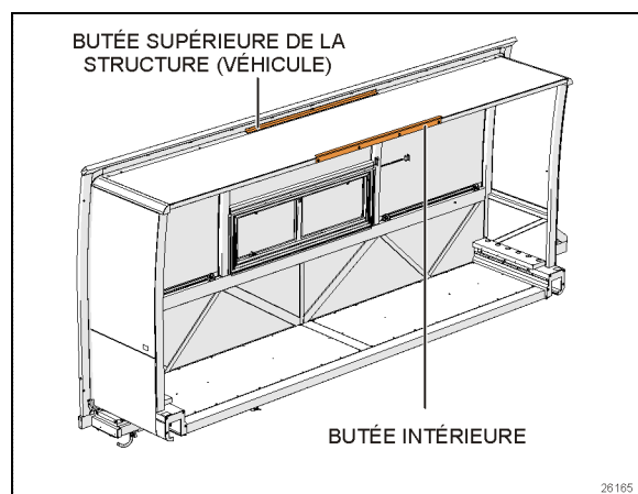
FIGURE 9: BUTÉE SUPÉRIEURE INTÉRIEURE
