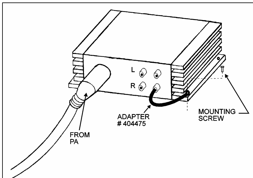
FIGURE 1: BLAUPUNKT AMPLIFIER
