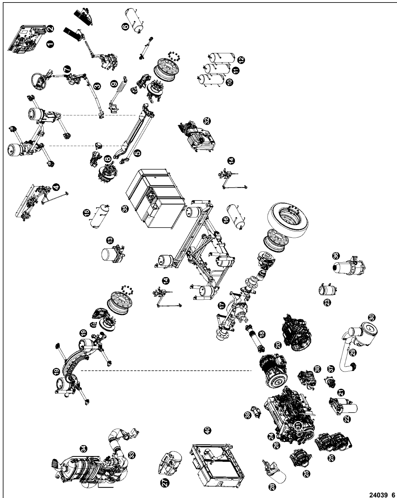
FIGURE 2: POINTS DE LUBRIFICATION ET D'ENTRETIEN (ESSIEU AVANT RIGIDE ILLUSTRÉ) TYPIQUES
