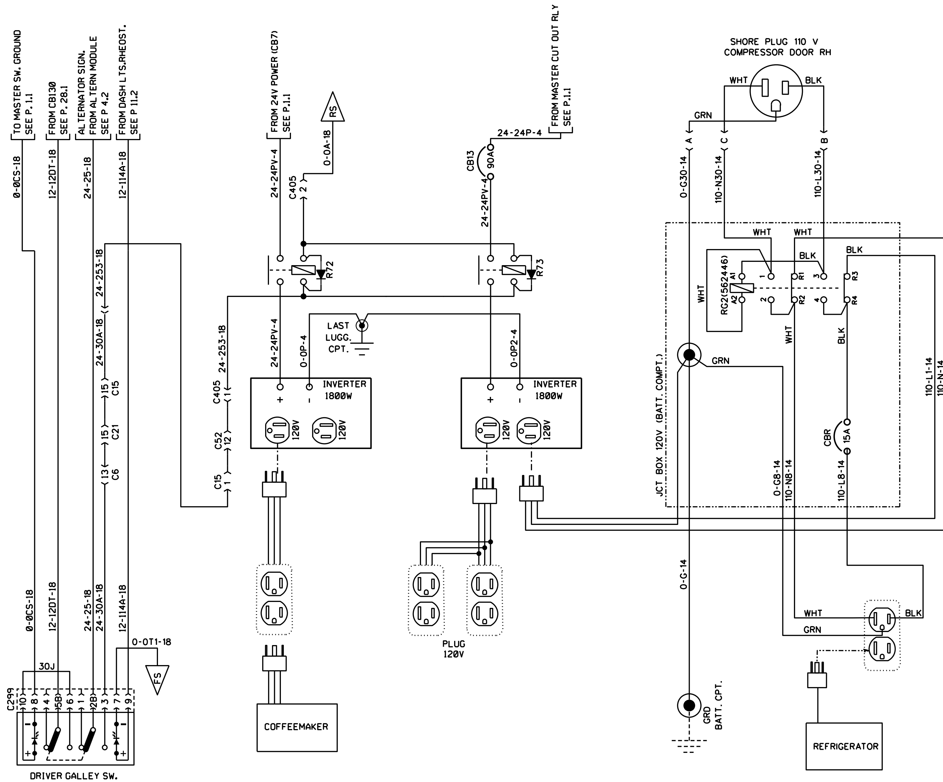
120V OUTLET
