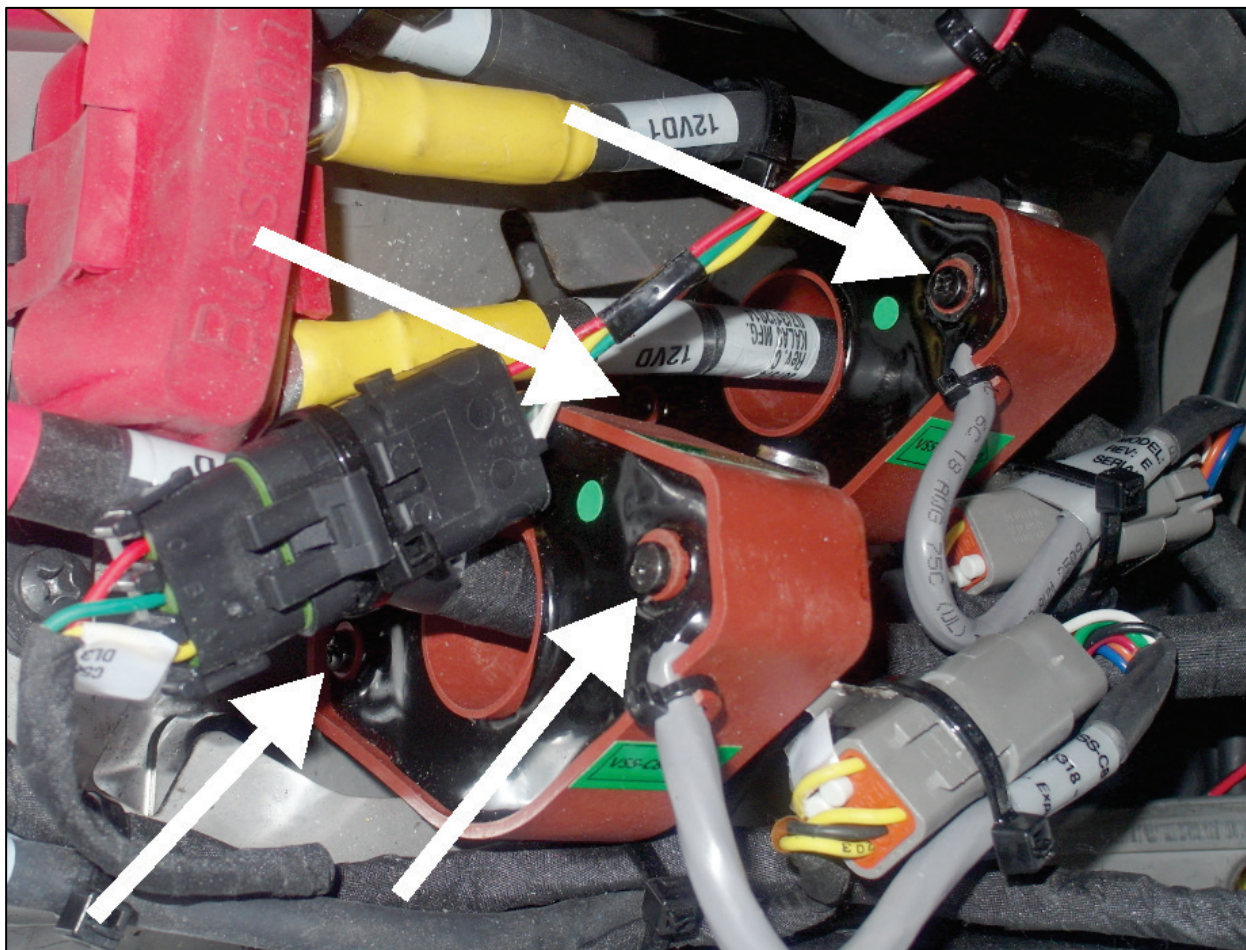
Figure 15 : Vis de montage, Série X
