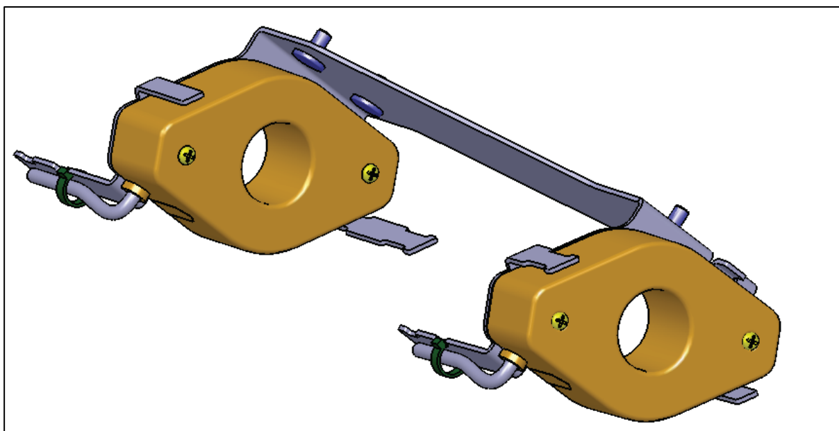
Figure 14 H Support des capteurs.
