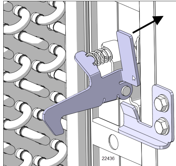
VERROU SECONDAIRE
