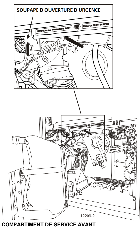
COMPARTIMENT DE SERVICE AVANT
