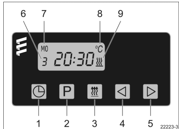
FIGURE 1: MINUTERIE DU PRÉCHAUFFEUR
