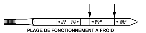
JAUGE DE L'HUILE À TRANSMISSION (TYPIQUE) 07050
