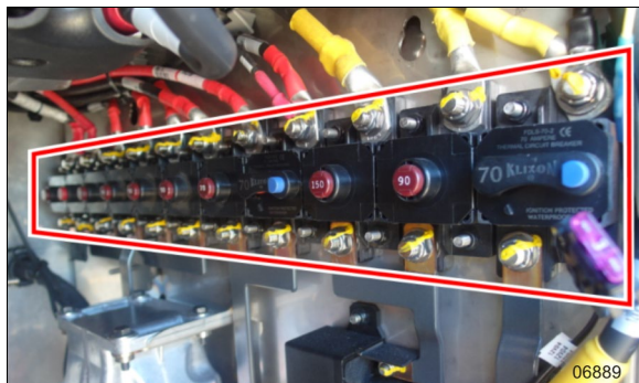
DISJONCTEURS PRINCIPAUX
