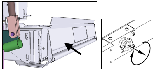
LEVAGE DU CADRE ET DU CHARRIOT À LA MÊME HAUTEUR
