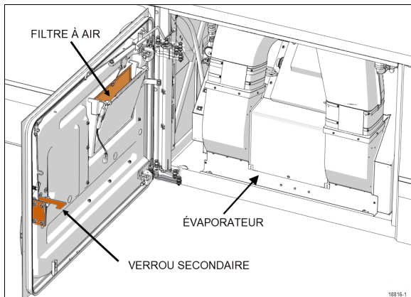
LEVIER DE DÉVERROUILLAGE SECONDAIRE
