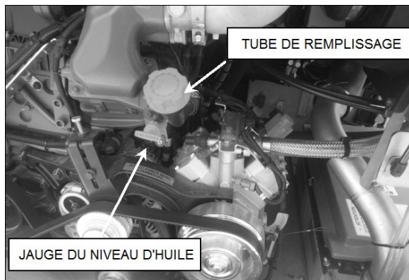
MOTEUR VOLVO D13
