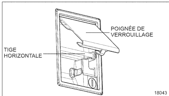
SERRURE ET POIGNÉE DE LA PORTE DES COMPARTIMENTS À BAGAGES 18043
