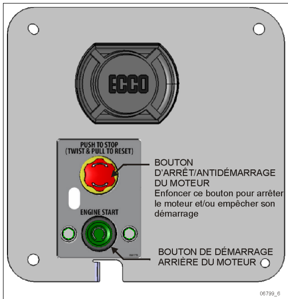
PANNEAU DE DÉMARRAGE ARRIÈRE
