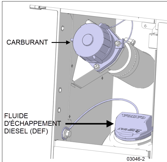
PORTE D'ACCÈS AU COL DE REMPLISSAGE DE CARBURANT ET DE DEF
