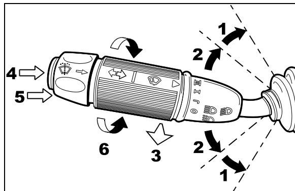
LEVIER À FONCTIONS MULTIPLES S23133
