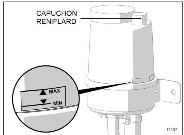
RÉSERVOIR DE FLUIDE DE LA DIRECTION ASSISTÉE
