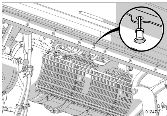
LOQUET DE LA PORTE D'ACCÈS
