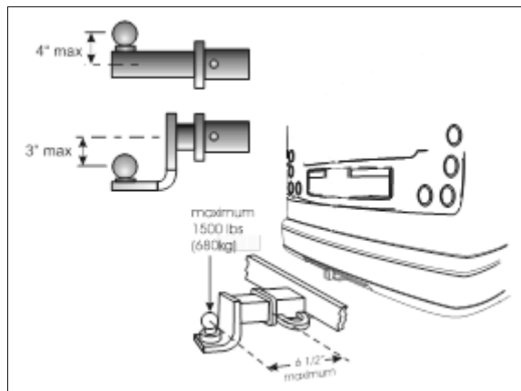
DISPOSITIF D'ATTELAGE
