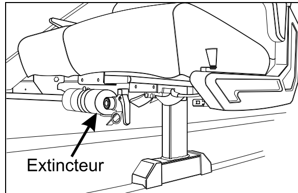
EMPLACEMENT DES EXTINCTEURS SOUS LES PREMIERS SIÈGES 23136
