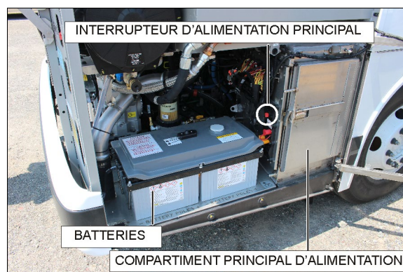
COMPARTIMENT À LA DROITE DU MOTEUR
