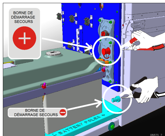
POSITION DES BORNES POUR DÉMARRAGE-SECOURS
