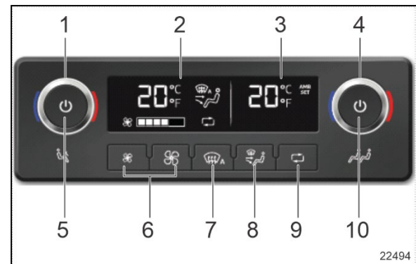
UNITÉ DE COMMANDE DU SYSTÈME CVC
