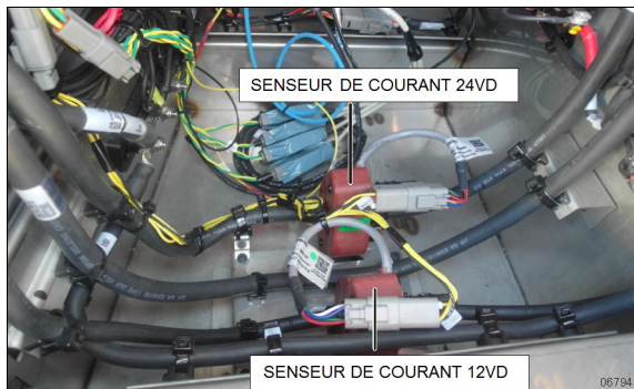
CAPTEURS DE COURANT 12VD & 24VD
