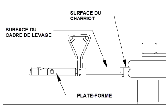
LEVAGE DU CADRE ET DU CHARRIOT À LA MÊME HAUTEUR
