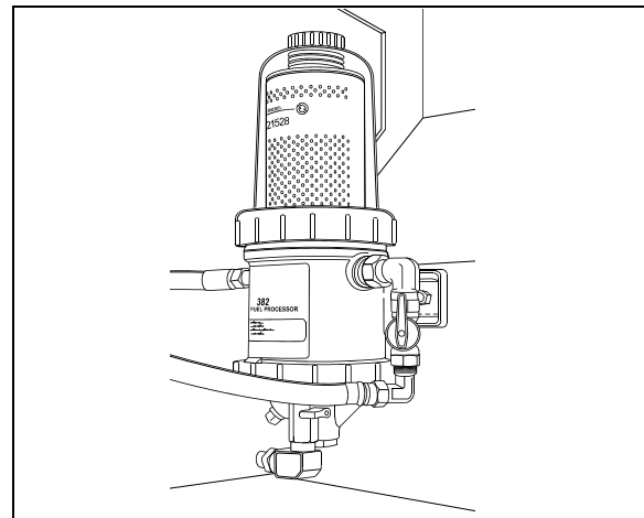
SYSTÈME DE FILTRATION DAVCO FUEL PRO 382
