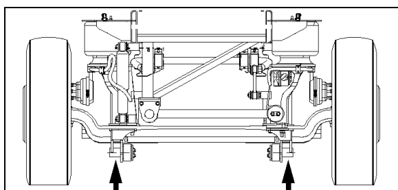
POINTS DE LEVAGE SOUS L'ESSIEU AVANT - ESSIEU RIGIDE
