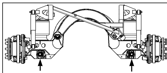
POINTS DE LEVAGE SOUS L'ESSIEU AUXILIAIRE
