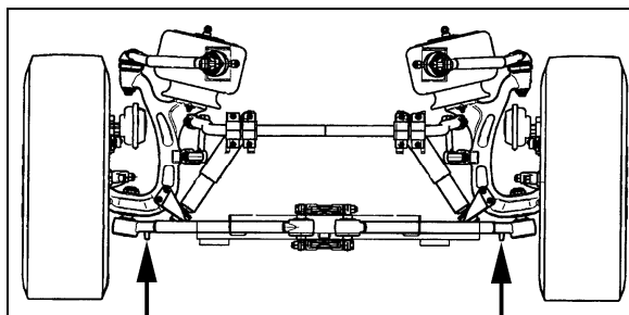
POINTS DE LEVAGE SOUS L'ESSIEU AVANT - SUSPENSION INDÉPENDANTE
