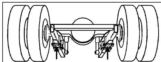
POINTS DE LEVAGE SOUS L'ESSIEU MOTEUR
