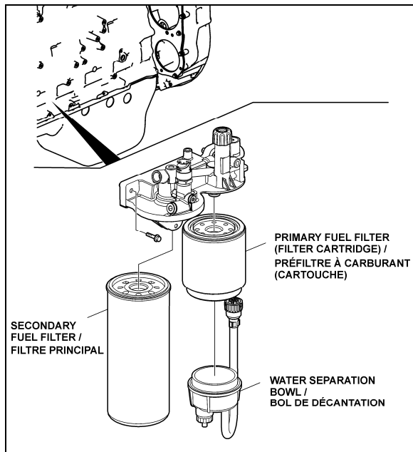
FILTRES À CARBURANT - MOTEUR VOLVO D13
