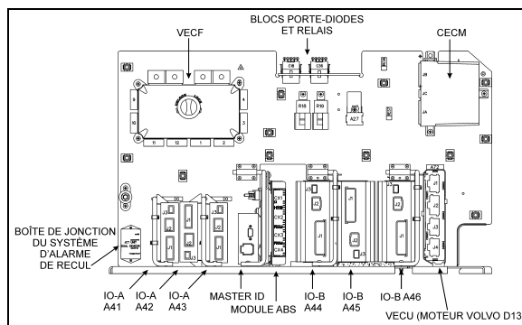
COMPARTIMENT ÉLECTRIQUE AVANT
