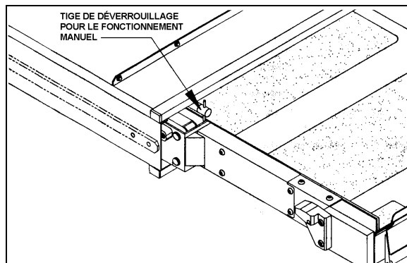
TIGES DE DÉVERROUILLAGE DE LA PLATE-FORME 23334
