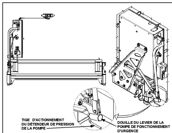
POMPE DE FONCTIONNEMENT D'URGENCE
