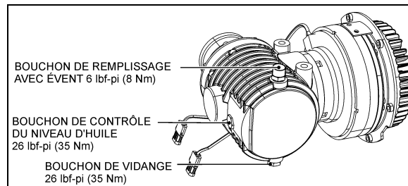
NIVEAU D'HUILE DE LA BOÎTE D'ENGRENAGES
