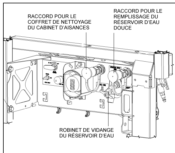
RACCORDS POUR L'ENTRETIEN DU RÉSERVOIR D'EAU DOUCE 12219_3
