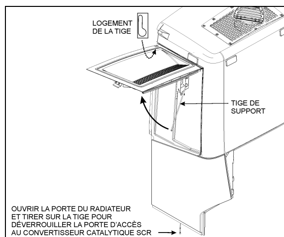
ACCÈS AU CONVERTISSEUR CATALYTIQUE SCR
