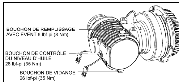
NIVEAU D'HUILE DE LA BOÎTE D'ENGRENAGES
