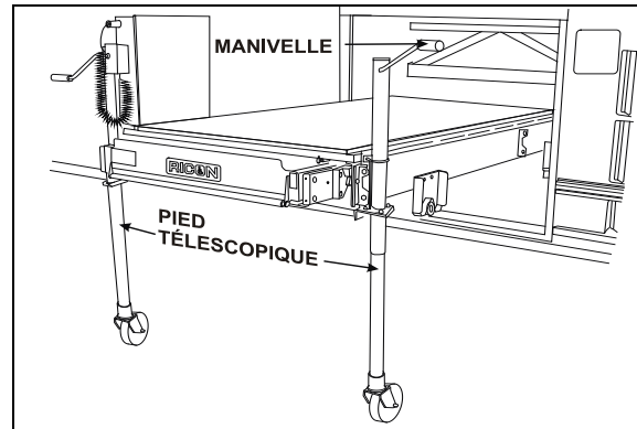
INSTALLATION DES PIEDS TÉLESCOPIQUES
