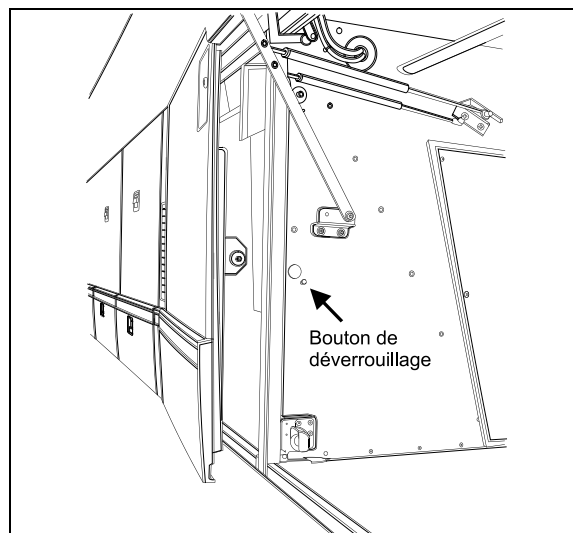
ACCÈS AU COMPARTIMENT DE L'ÉVAPORATEUR
