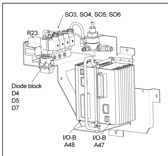
PANNEAU D'ACCESSOIRES PNEUMATIQUES DE LA CONSOLE DE DROITE 06596
