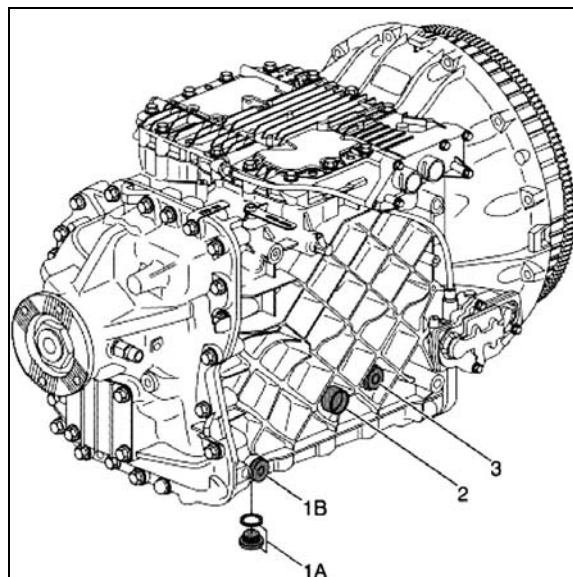
ORIFICE DE REMPLISSAGE TRANSMISSION I-SHIFT 07111
