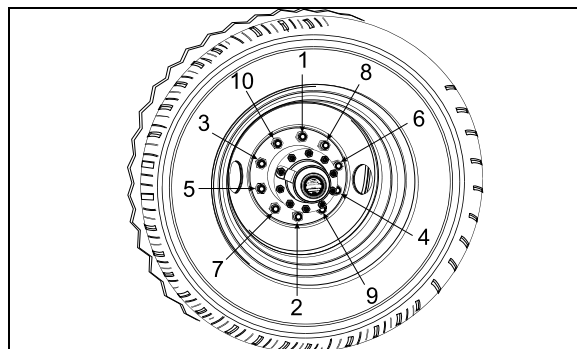
ORDRE DE SERRAGE
