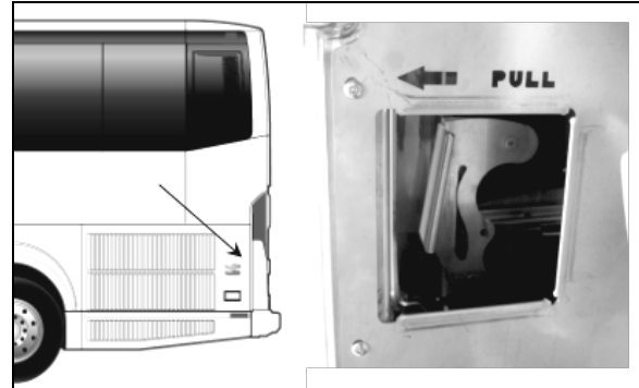
POSITION DU LOQUET PORTE DU RADIATEUR 18529_2
