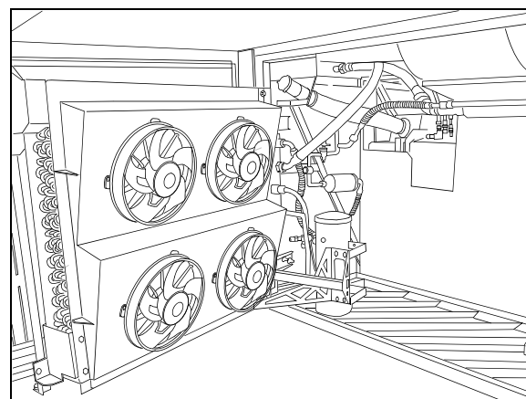
COMPARTIMENT DU CONDENSEUR 22362
