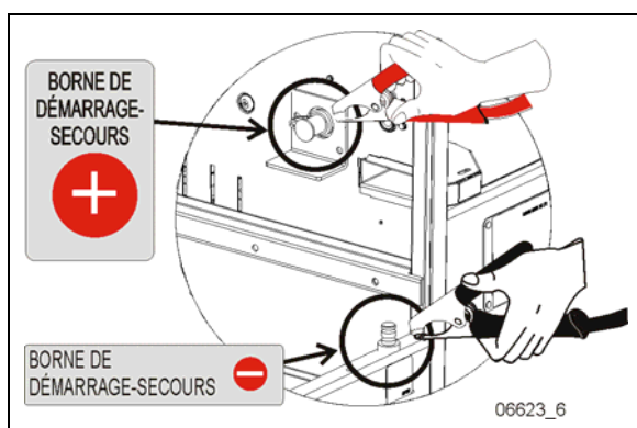
BORNES DE DÉMARRAGE-SECOURS
