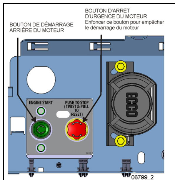
PANNEAU DU DÉMARRAGE ARRIÈRE DU MOTEUR
