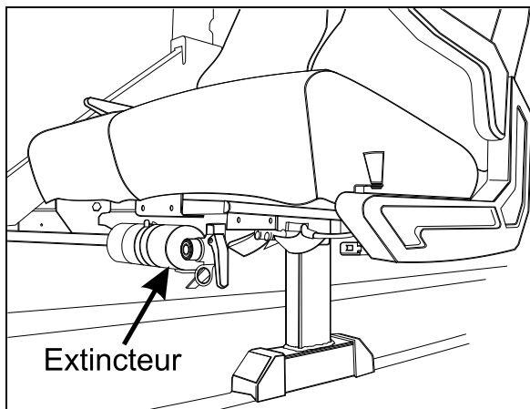
EMPLACEMENT DES EXTINCTEURS SOUS LES PREMIERS SIÈGES 23136
