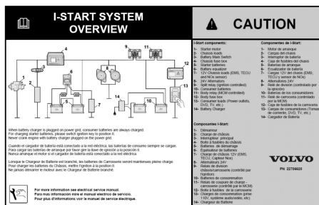
Autocollant de description du système I-Start.
