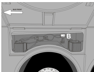
(B) Mini porte-fusibles à l'intérieur du compartiment à batteries gauche.
