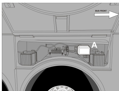
(A) Boîte à fusibles et relais du châssis à l'intérieur du compartiment de batteries droit.
