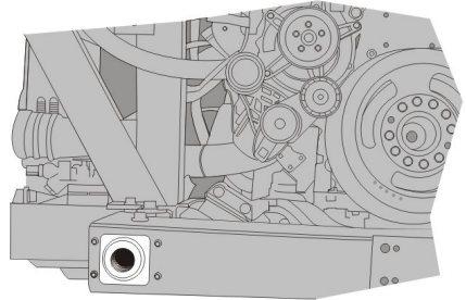
Endroit pour la fixation de barre de remorquage (avant).
