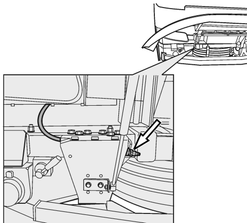
Emplacement du raccord d'alimentation en air avant
