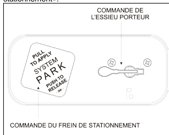
COMMANDE DE L'ESSIEU AUXILIAIRE ET FREIN DE STATIONNEMENT 12129_FR
