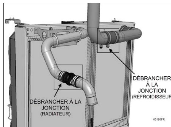
FIGURE 38: CONNEXIONS SUP. DU RADIATEUR & DU REFROIDISSEUR D'AIR (CAC)
