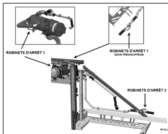
FIGURE 21: ROBINETS DU SYSTÈME DE CHAUFFAGE
