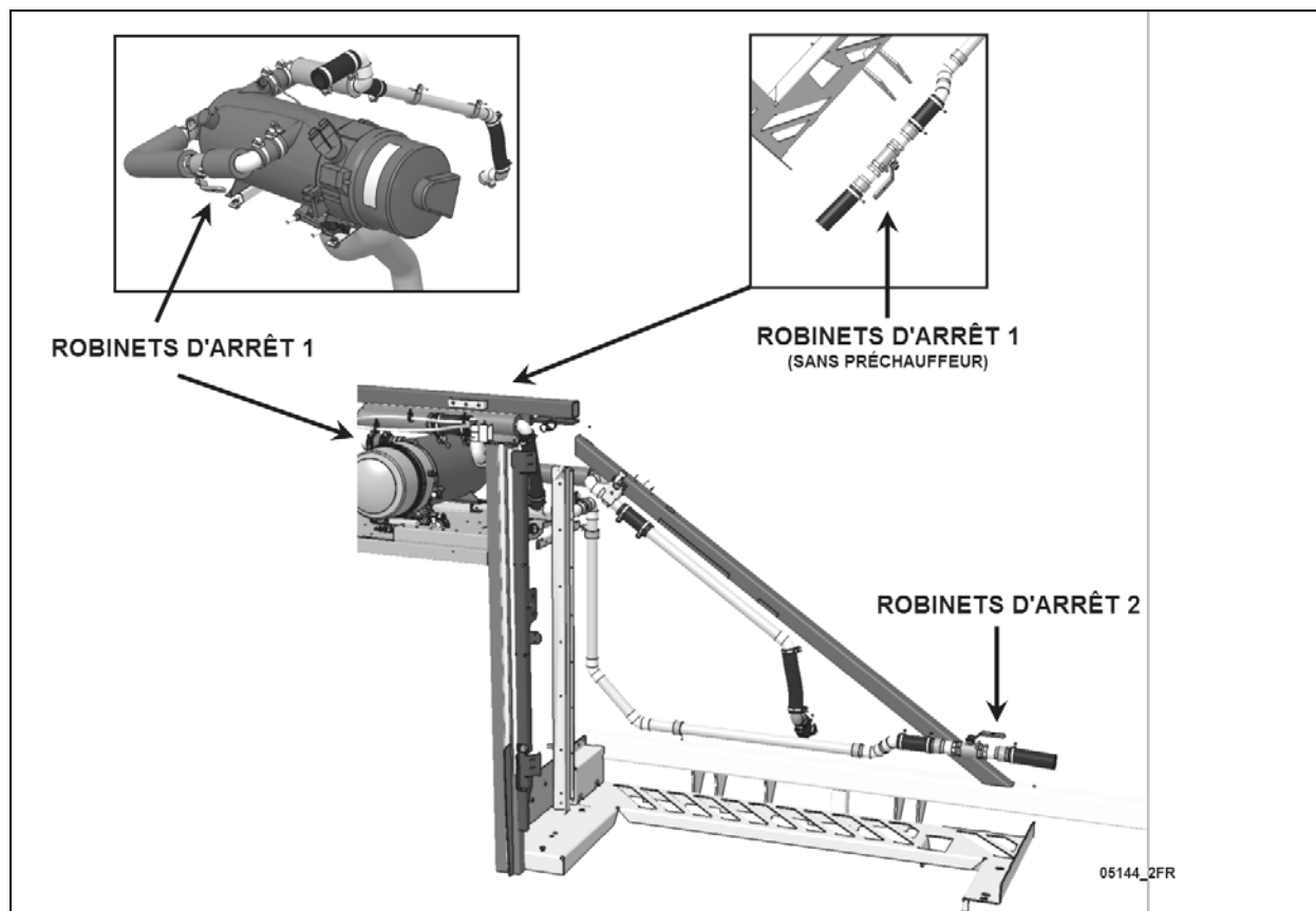
FIGURE 10 : ROBINETS D'ARRÊT DE CANALISATIONS DE CHAUFFAGE - COMPARTIMENT MOTEUR SERIE H3
