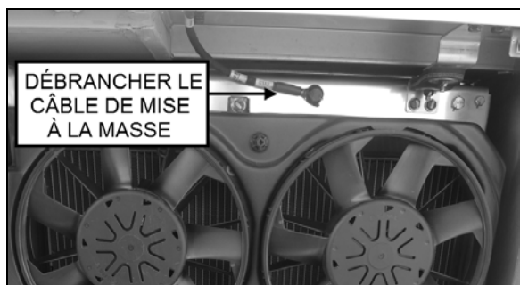
FIGURE 40: CÂBLE DE MISE À LA MASSE DU SYSTÈME DE REFROIDISSEMENT
