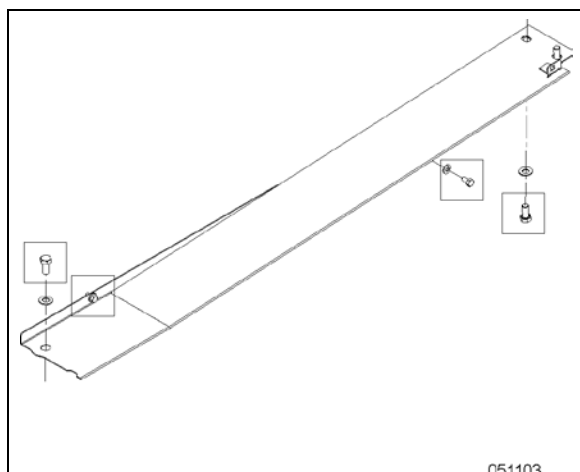
FIGURE 27: VIS DE MONTAGE DU PROTECTEUR ANTI-ÉCLABOUSSURE
