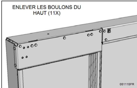
FIGURE 54: VIS DE LA SECTION AVANT SUPÉRIEURE
