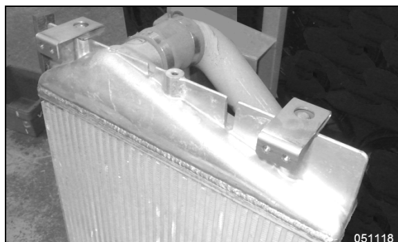
FIGURE 58: ÉQUERRES DE SUPPORT ET TUYAU SUPÉRIEUR DU REFROIDISSEUR D'AIR (CAC)
