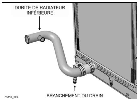
FIGURE 22: CONNEXION POUR LA VIDANGE DU LIQUIDE DE REFROIDISSEMENT
