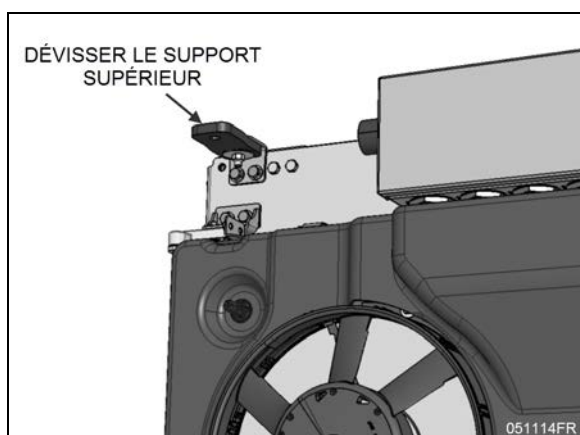
FIGURE 52: SUPPORT SUPÉRIEUR (CÔTÉ REFROIDISSEUR D'AIR)
