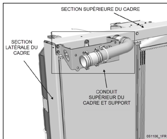
FIGURE 30: ÉLÉMENTS À DÉMONTER POUR LE REMPLACEMENT DU RADIATEUR
