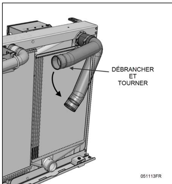
FIGURE 51: TUYAU SUPÉRIEUR DU REFROIDISSEUR D'AIR (CAC) SUR SÉRIE X3 SEULEMENT
