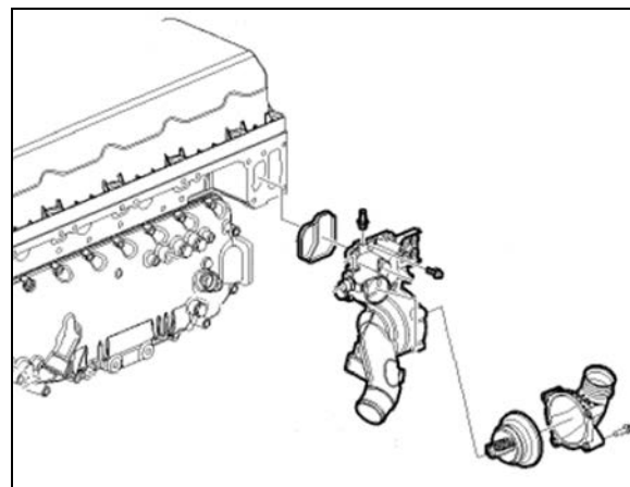
FIGURE 8 : BOÎTIER DU THERMOSTAT - VOLVO D13
