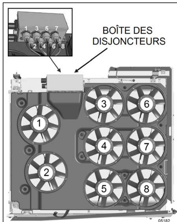
FIGURE 13: NUMÉRO D'IDENTIFICATION DES VENTILATEURS ET DES CONNECTEURS SOUS LA BOÎTE DE DISJONCTEURS
