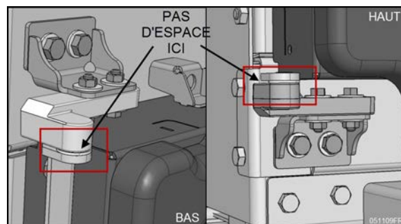
FIGURE 32: INSTALLATION DES CHARNIÈRES DU CARÉNAGE DE VENTILATEURS
