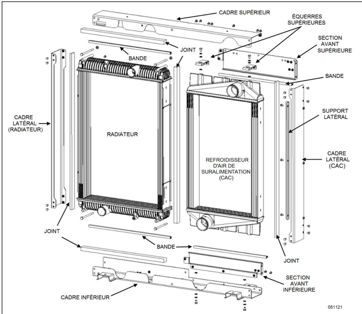
FIGURE 53: VUE ÉCLATÉE DU MODULE DE REFROIDISSEMENT
