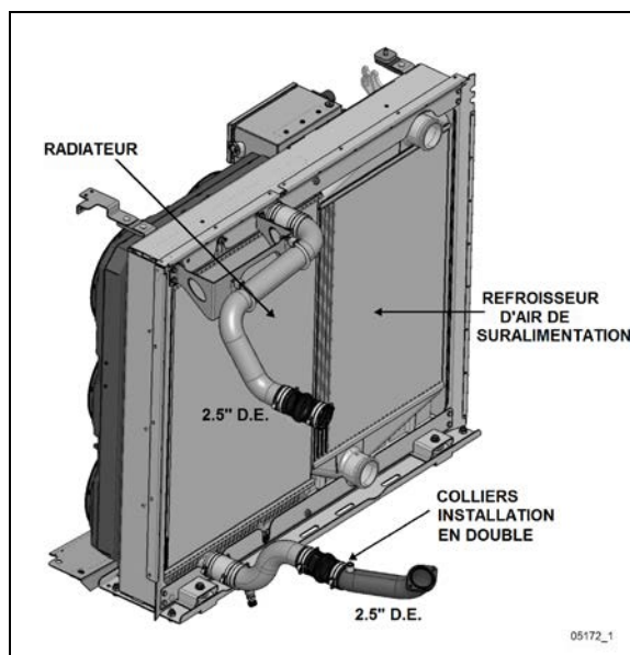
FIGURE 4: CIRCULATION DU LIQUIDE DE REFROIDISSEMENT (SÉRIE X3)
