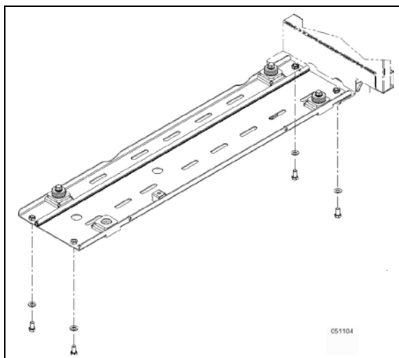
FIGURE 28: VIS DE MONTAGE DU SUPPORT INFÉRIEUR
