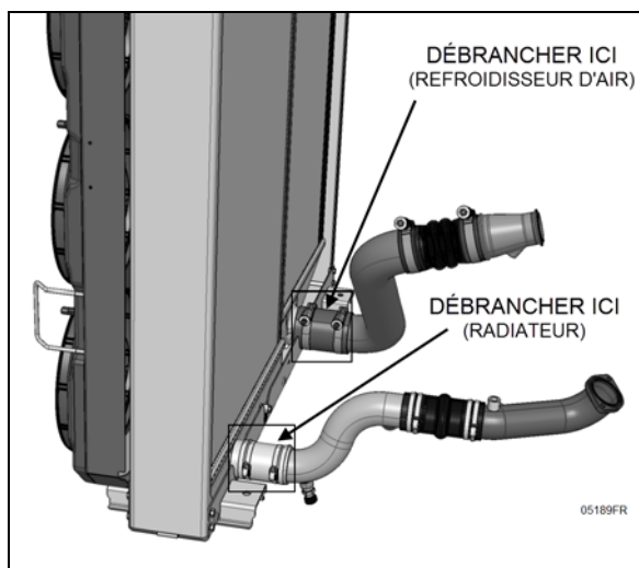
FIGURE 39: CONNEXIONS INF. DU RADIATEUR & DU REFROIDISSEUR D'AIR (CAC)
