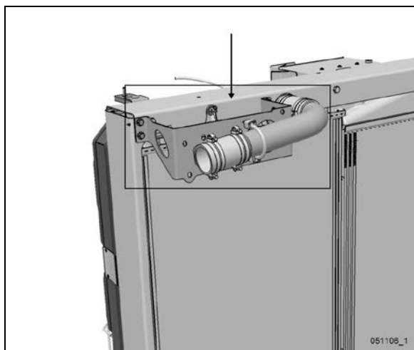
FIGURE 34: INSTALLATION DU TUYAU, SUPPORT ET ATTACHES DU RADIATEUR
