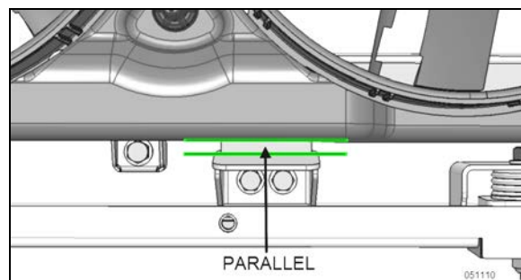
FIGURE 33: AJUSTEMENT DU BAS DU CARÉNAGE AVEC LE SUPPORT INFÉRIEUR
