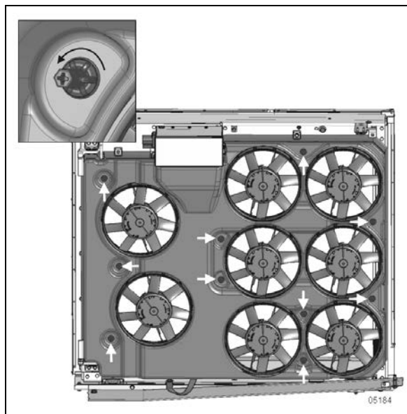
FIGURE 15: POSITION DES ATTACHES DU COUVERCLE DE PROTECTION
