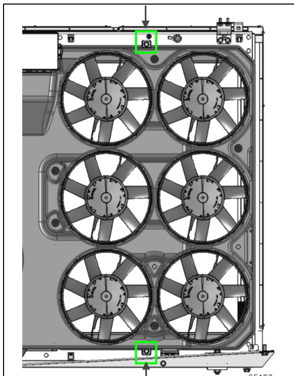
FIGURE 18: VIS INFÉRIEURE ET SUPÉRIEURE DU CARÉNAGE DE VENTILATEURS
