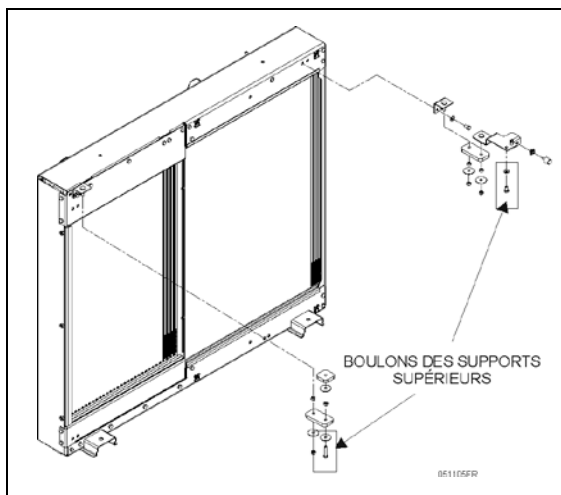
FIGURE 29: VIS DE MONTAGE DES SUPPORTS SUPÉRIEURS
