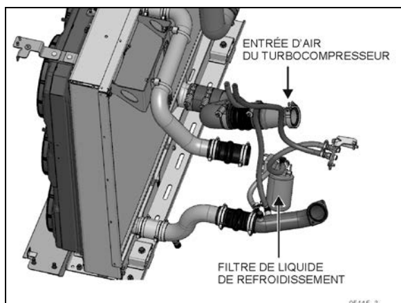
FIGURE 12 : FILTRE DU LIQUIDE DE REFROIDISSEMENT (SÉRIE X3 MONTRÉE)
