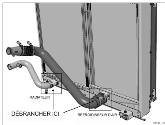
FIGURE 24: CONNEXIONS INF. DU RADIATEUR & DU REFROIDISSEUR D'AIR (CAC)
