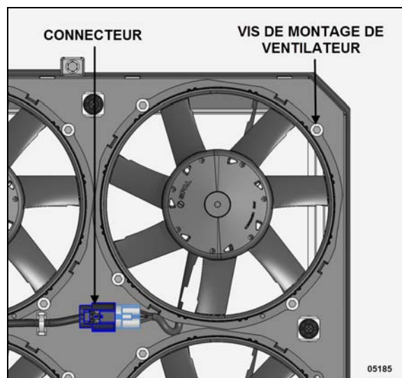
FIGURE 16: POSITION DU CONNECTEUR ET DES VIS DE MONTAGE
