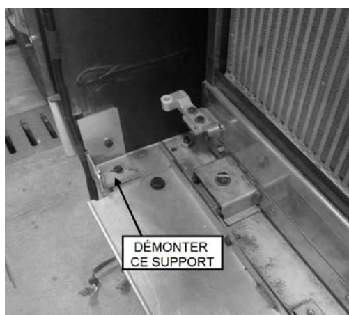
FIGURE 42: SUPPORT DE CHARNIÈRE INFÉRIEURE DE LA PORTE DU RADIATEUR
