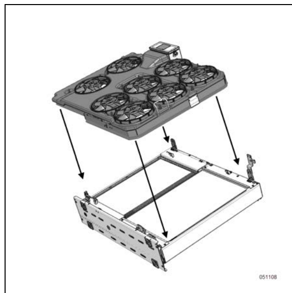
FIGURE 47: POSITIONNEMENT DU CARÉNAGE DE VENTILATEURS
