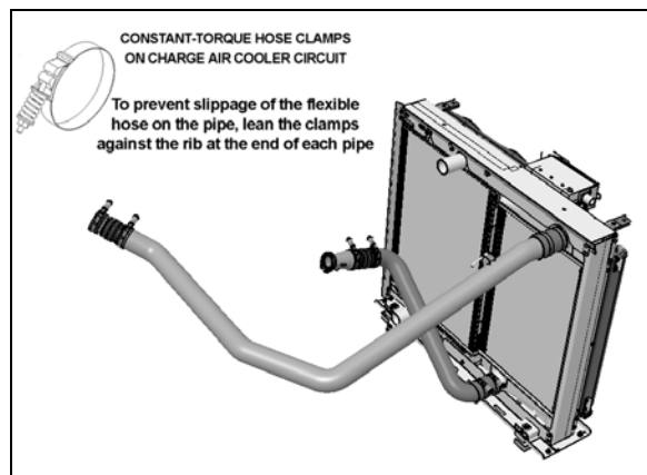
FIGURE 7 : COLLIERS DE SERRAGE DU REFROIDISSEUR D'AIR DE SURALIMENTATION (SÉRIE H3)
