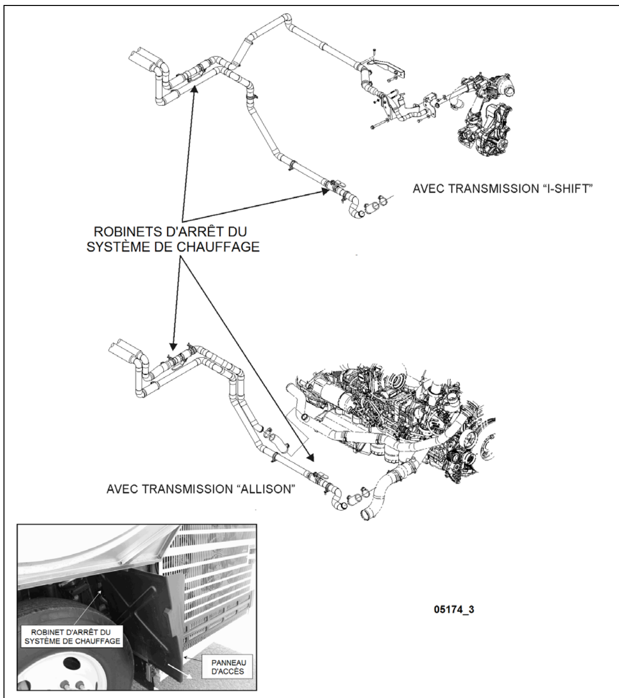
FIGURE 9 : ROBINETS D'ARRÊT DE CANALISATIONS DE CHAUFFAGE - COMPARTIMENT MOTEUR SÉRIE X3
