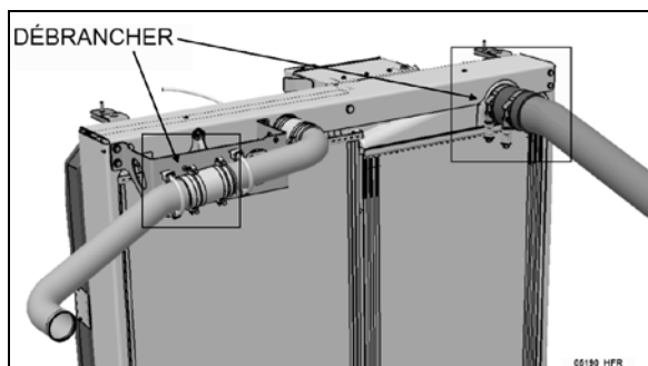
FIGURE 23: CONNEXIONS SUP. DU RADIATEUR & DU REFROIDISSEUR D'AIR (CAC)
