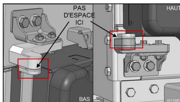
FIGURE 48: INSTALLATION DES CHARNIÈRES DU CARÉNAGE DE VENTILATEURS
