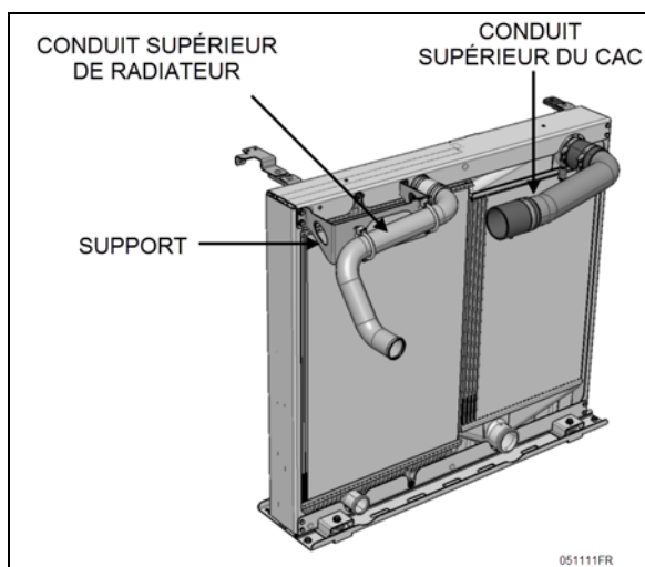
FIGURE 50: INSTALLATION DES TUYAUX, SUPPORTS ET ATTACHES DU REFROIDISSEUR D'AIR ET DU RADIATEUR
