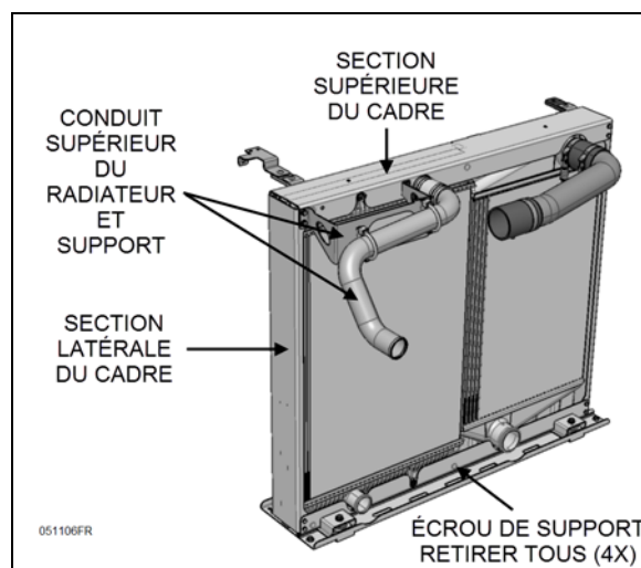
FIGURE 46: ÉLÉMENTS À DÉMONTER POUR LE REMPLACEMENT DU RADIATEUR
