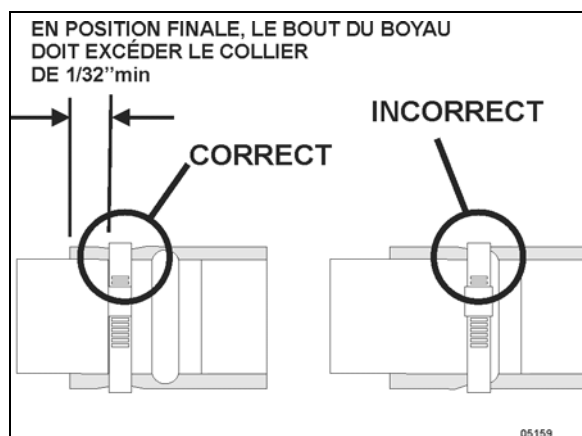
FIGURE 6: INSTALLATION CORRECTE DES COLLIERS DE SERRAGE
