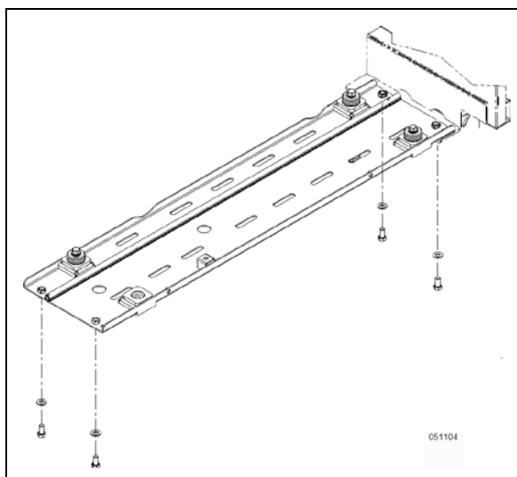
FIGURE 44: VIS DE MONTAGE DU SUPPORT INFÉRIEUR
