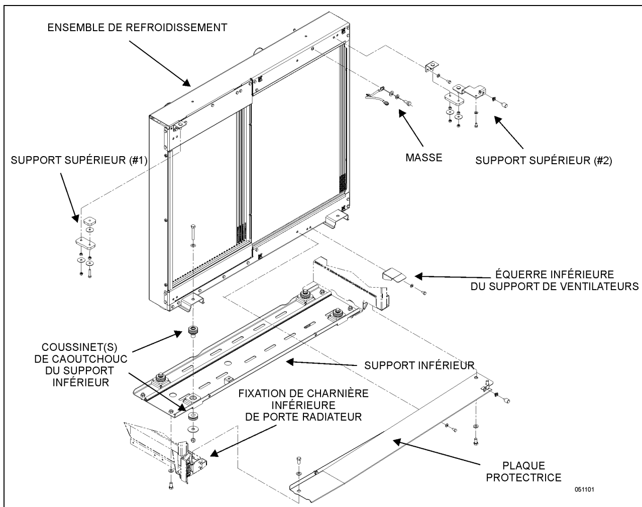
FIGURE 41: COMPOSANTS ET SUPPORTS DU MODULE DE REFROIDISSEMENT
