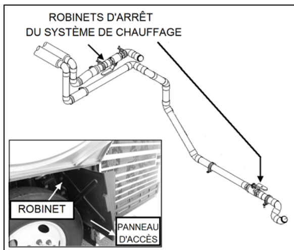
FIGURE 36: ROBINETS DU SYSTÈME DE CHAUFFAGE
