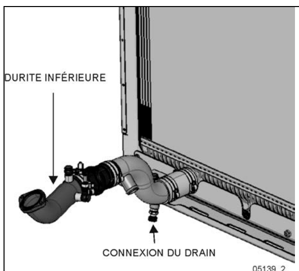
FIGURE 37: CONNEXION POUR LA VIDANGE DU LIQUIDE DE REFROIDISSEMENT
