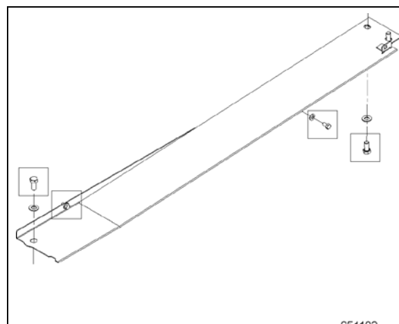
FIGURE 43: VIS DE MONTAGE DU PROTECTEUR ANTI-ÉCLABOUSSURE
