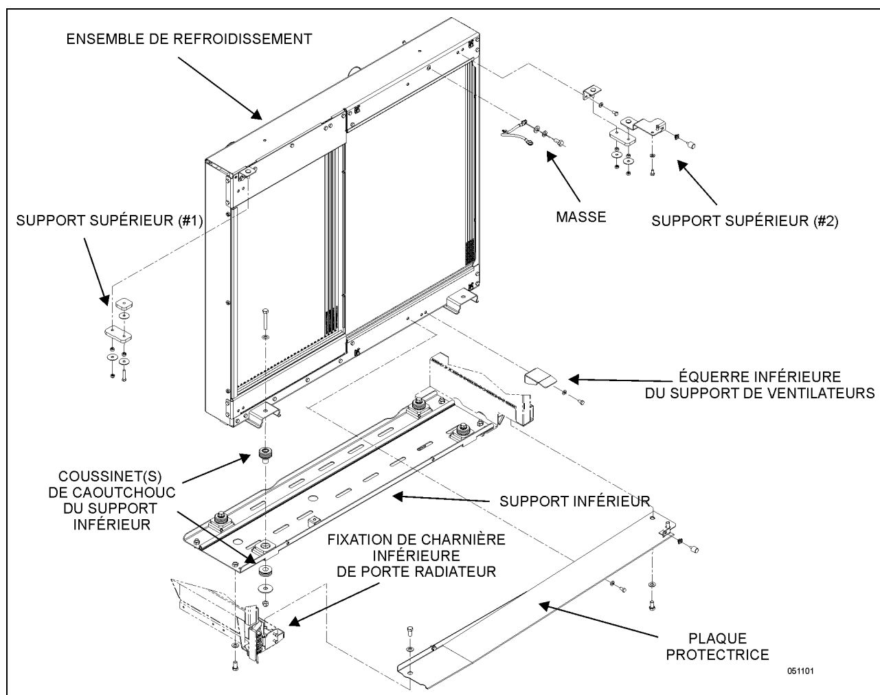
FIGURE 26: COMPOSANTS ET SUPPORTS DU MODULE DE REFROIDISSEMENT
