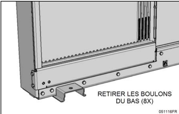
FIGURE 55: VIS DE LA SECTION AVANT INFÉRIEURE
