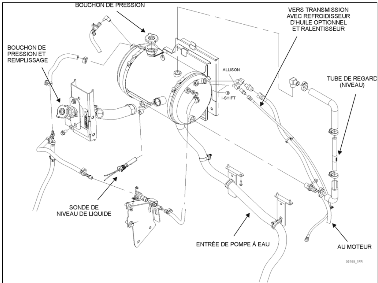
FIGURE 3 : RÉSERVOIR D'EXPANSION DU LIQUIDE DE REFOUÏSSEMENT SUR LA SÉRIE H3
