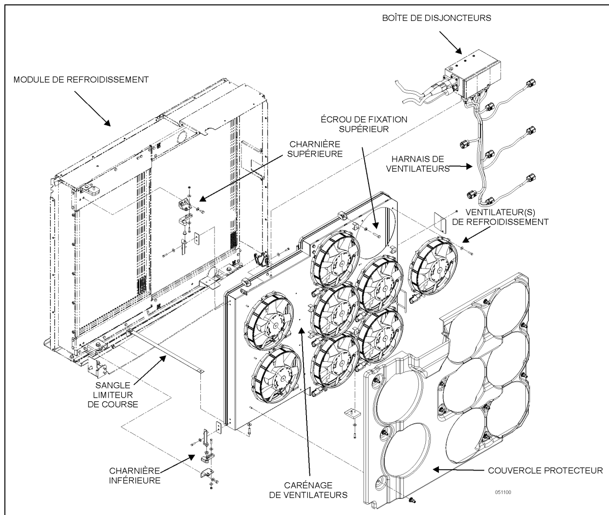
FIGURE 14: PRINCIPAUX COMPOSANTS DE L'ASSEMBLAGE DU SYSTÈME DE REFROIDISSEMENT
