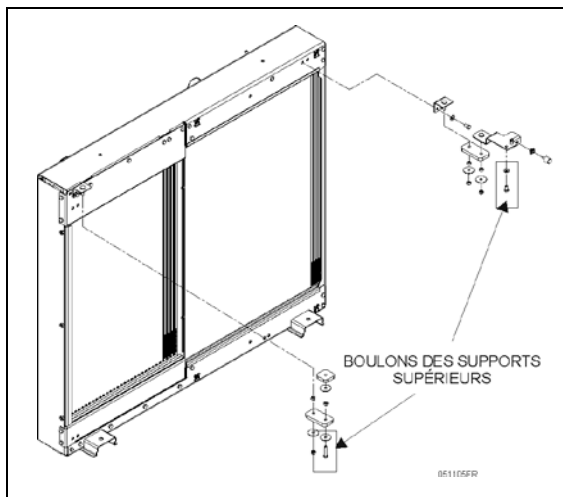
FIGURE 45: VIS DE MONTAGE DES SUPPORTS SUPÉRIEURS
