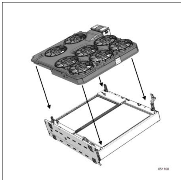
FIGURE 31: POSITIONNEMENT DU CARÉNAGE DE VENTILATEURS
