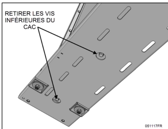
FIGURE 57: VIS DU DESSOUS DU REFROIDISSEUR D'AIR (CAC)
