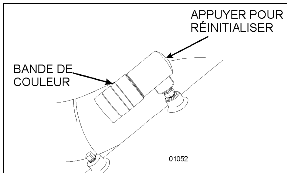
FIGURE 33 : INDICATEUR D'OBSTRUCTION
