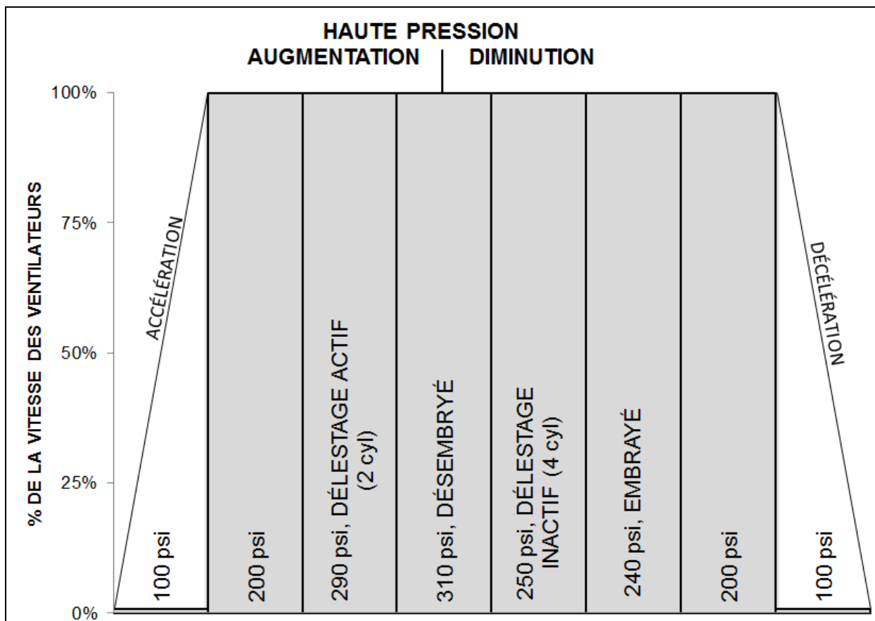
FIGURE 42: VITESSE DES VENTILATEURS DU CONDENSEUR ET ÉVÈNEMENTS AU COMPRESSEUR SELON LA PRESSION DU CÔTÉ ÉLEVÉ.
