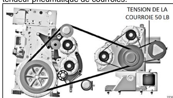
FIGURE 82: DISPOSITION DES COURROIES AVEC PETIT COMPRESSEUR DE CLIMATISATION SÉRIE X
