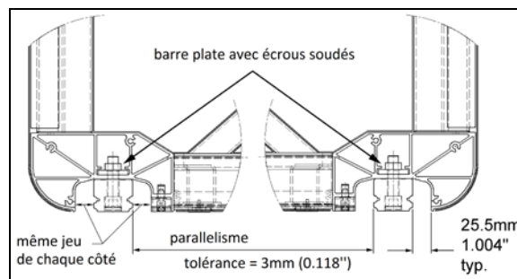
FIGURE 28: MISE EN PLACE DE RAIL 26159
