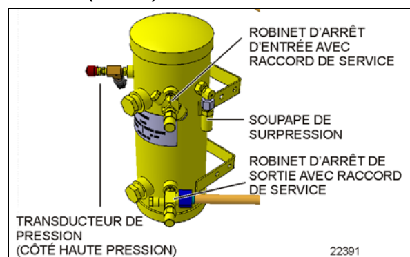
FIGURE 46: RÉSERVOIR DE RÉSERVE SÉRIE X
