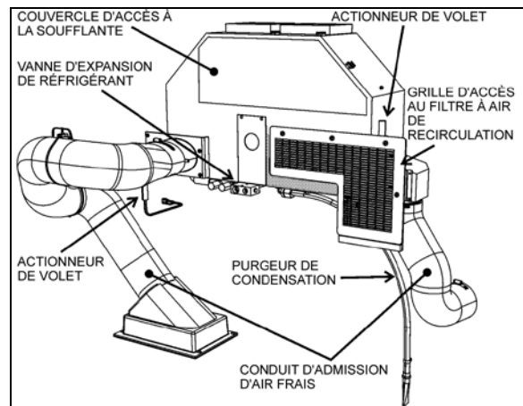
FIGURE 73 : UNITÉ DE CVC DU CONDUCTEUR
