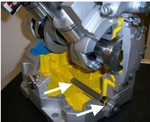
FIGURE 34: VUE EN COUPE MONTRANT LE FILTRE/CRÉPINE D'HUILE ET LE BOUCHON MAGNÉTIQUE DE VIDANGE
