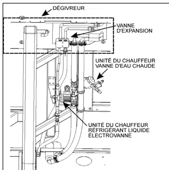
FIGURE 51 : ÉLECTROVANNE DU FLUIDE FRIGORIGÈNE DE L'UNITÉ DU CONDUCTEUR
