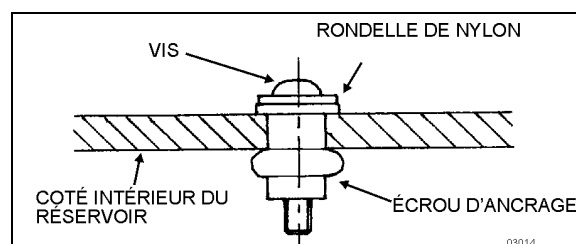
FIGURE 14 : RÉPARATION DU RÉSERVOIR DE CARBURANT
