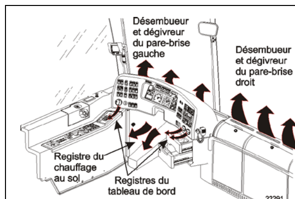
FIGURE 85 : CIRCULATION DE L'AIR DE L'UNITÉ DE CONDUCTEUR
