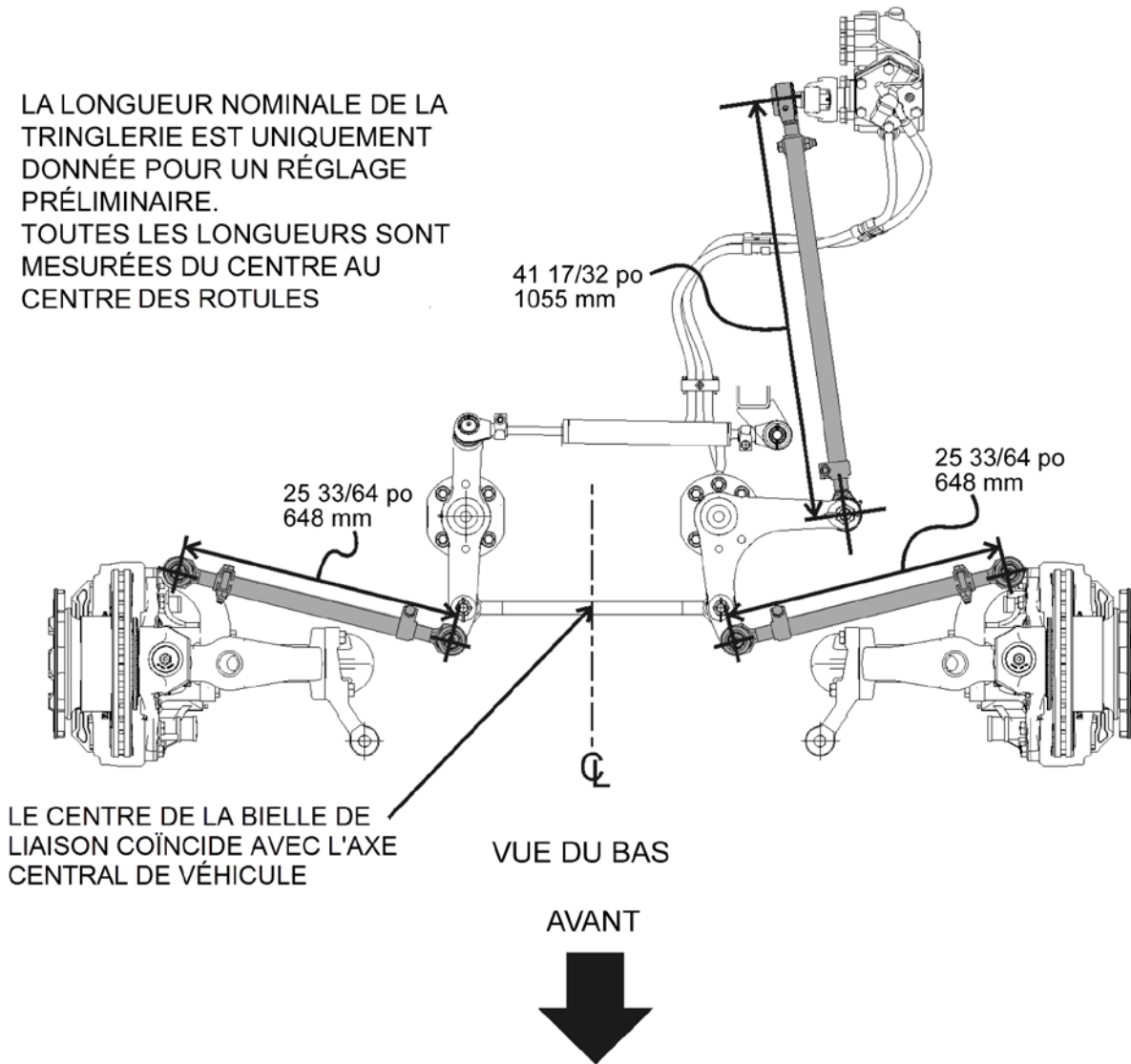
FIGURE 19: LONGUEURS NOMINALES DE TRINGLERIE DE DIRECTION
