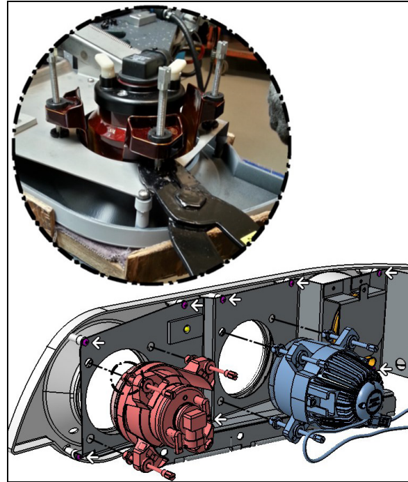
FIGURE 71: DÉTACHER LES EMBOUTS EN PLASTIQUE
