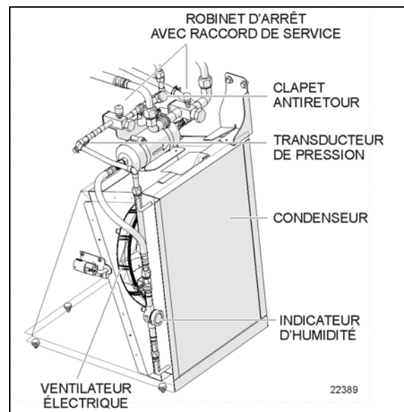
FIGURE 44 : ENSEMBLE DE CONDENSEUR DE PETIT SYSTÈME DE CLIMATISATION DE LA SÉRIE X
