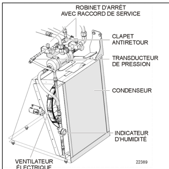
FIGURE 84: CONFIGURATION DE CONDENSEUR X3-45 VIP
