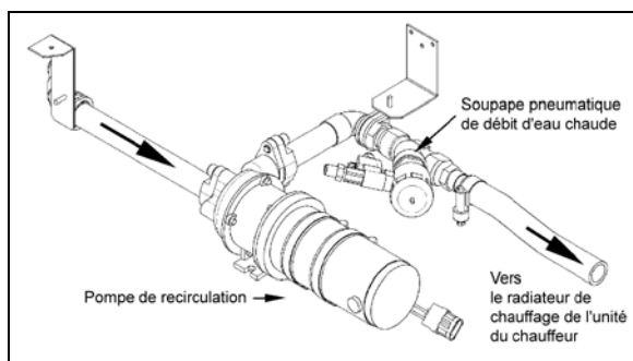
FIGURE 61: INSTALLATION DE LA POMPE DE CIRCULATION D'EAU CHAUDE (PETIT SYSTÈME DE CVC) 22292
