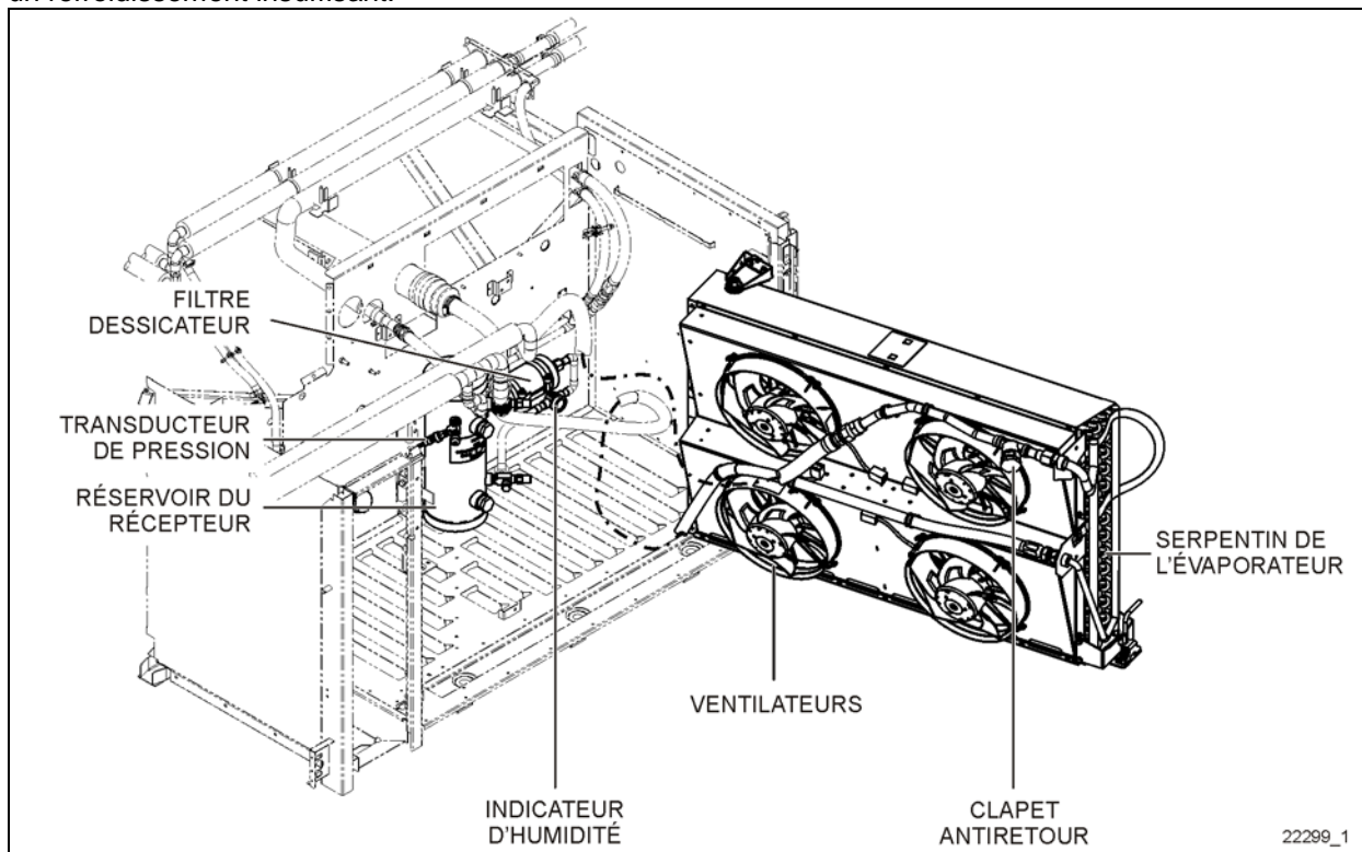
FIGURE 41: CONDENSEUR DE CLIMATISATION CENTRALE
