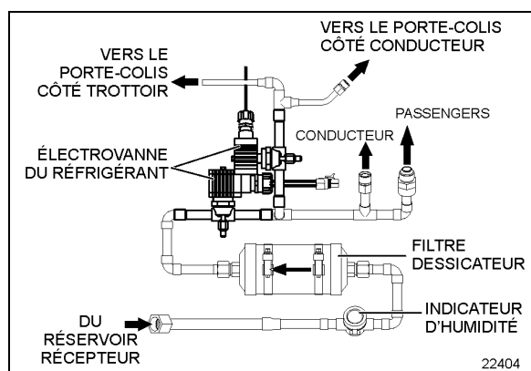
FIGURE 52 : ÉLECTROVANNE DE RÉFRIGÉRANT LIQUIDE DANS LE COMPARTIMENT DE CONDENSEUR (SÉRIE X)
