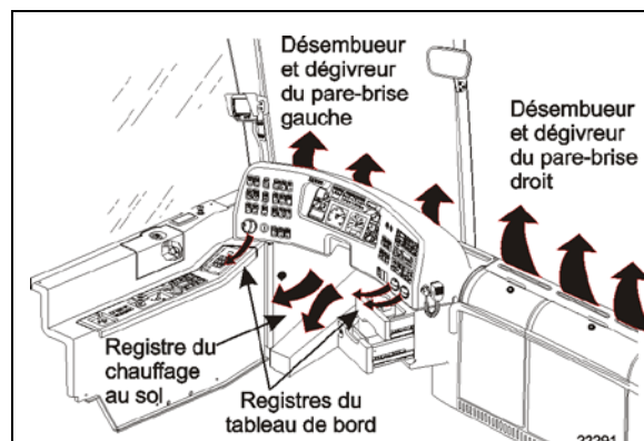
FIGURE 65 : CIRCULATION DE L'AIR DE L'UNITÉ DE CONDUCTEUR
