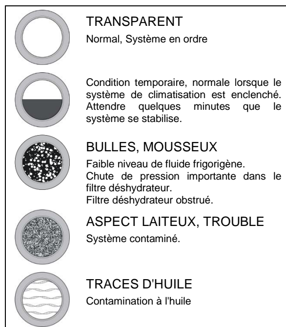
FIGURE 48 : CONDITIONS POUVANT ÊTRE OBSERVÉES DANS L'INDICATEUR D'HUMIDITÉ
