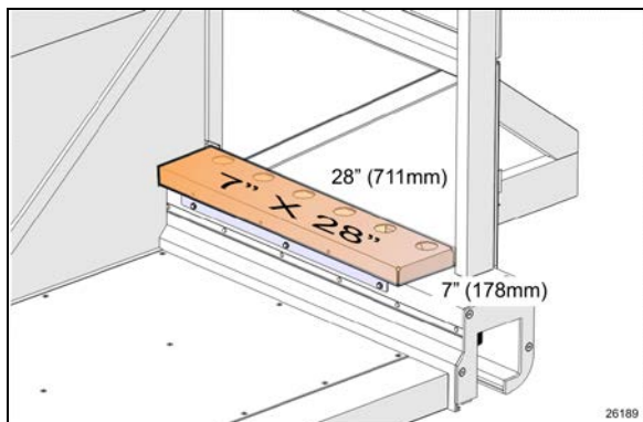
FIGURE 51: ZONE DE PERÇAGE INTERDIT, RALLONGE AVANT DROITE
