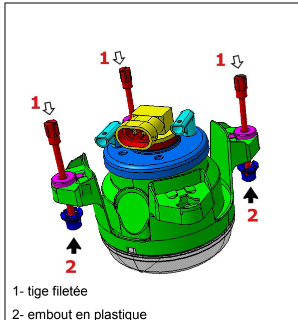
FIGURE 72: PROJECTEUR
