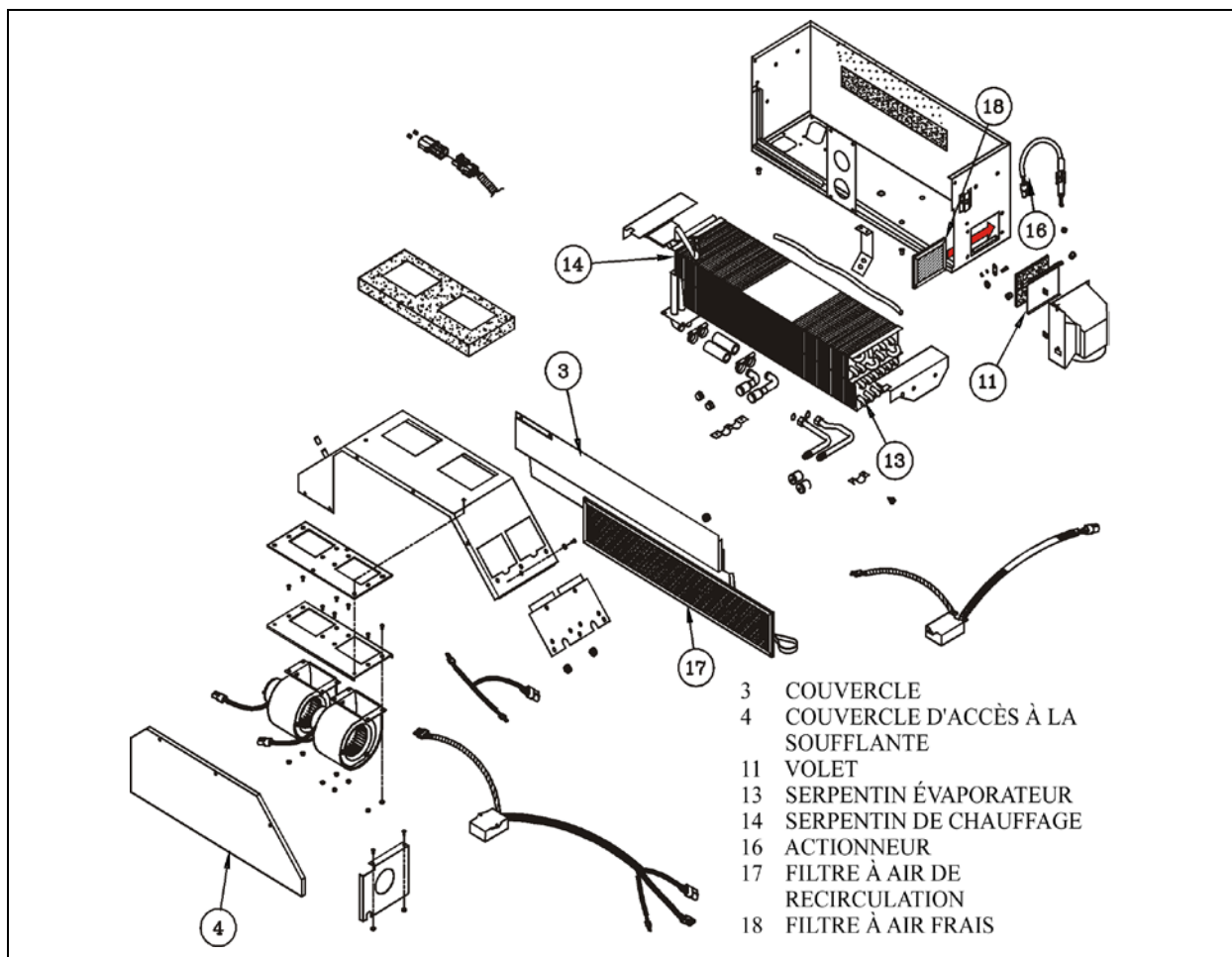
FIGURE 74 : UNITÉ DE CVC DU CONDUCTEUR
