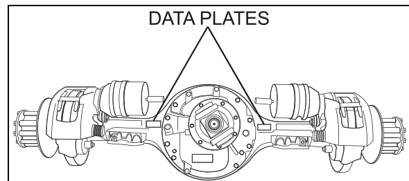
FIGURE 4: EMPLACEMENT PLAQUE SIGNALÉTIQUE AVEC NO. DE MODÈLE, NO. DE SÉRIE ET RAPPORT 00007
