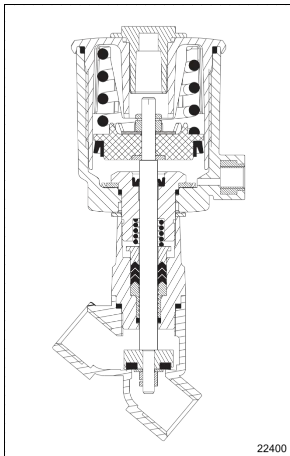
FIGURE 57: SOUPAPE PNEUMATIQUE D'EAU CHAUDE DE L'UNITÉ DE PASSAGER – VUE EN COUPE TYPE
