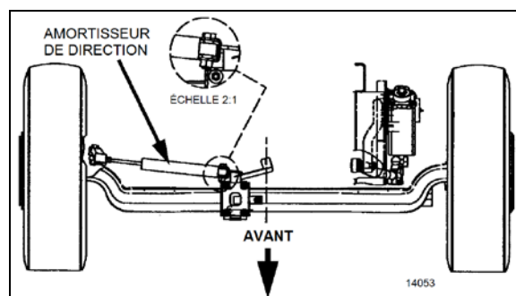
FIGURE 26 : STABILISATEUR DE DIRECTION (AMORTISSEUR)
