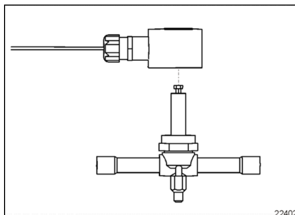
FIGURE 53 : ÉLECTROVANNE DE FLUIDE FRIGORIGÈNE TYPIQUE
