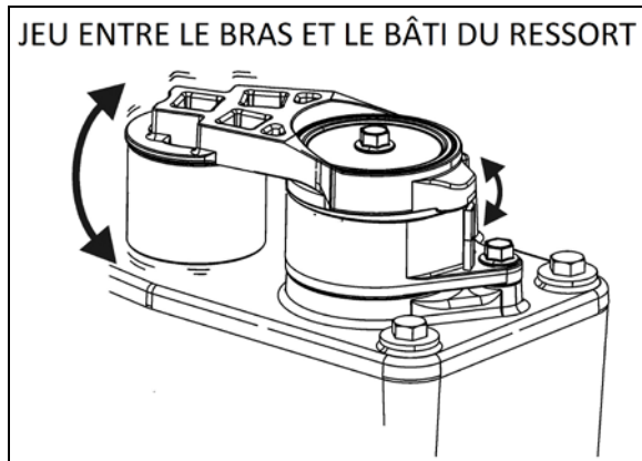
FIGURE 22 : VÉRIFICATION DE L'USURE DE LA BAGUE
