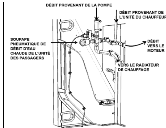
FIGURE 70: SOUPE PNEUMATIQUE DE DÉBIT D'EAU CHAUDE DE L'UNITÉ DES PASSAGERS
