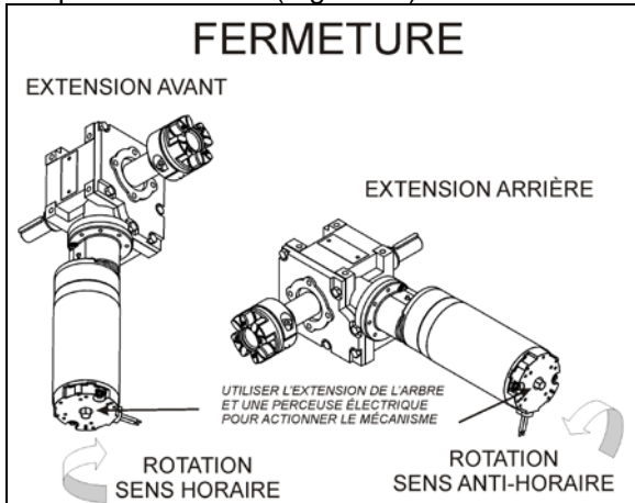
FIGURE 41: ROTATION DU MOTEUR DE LA RALLONGE COULISSANTE 26038
