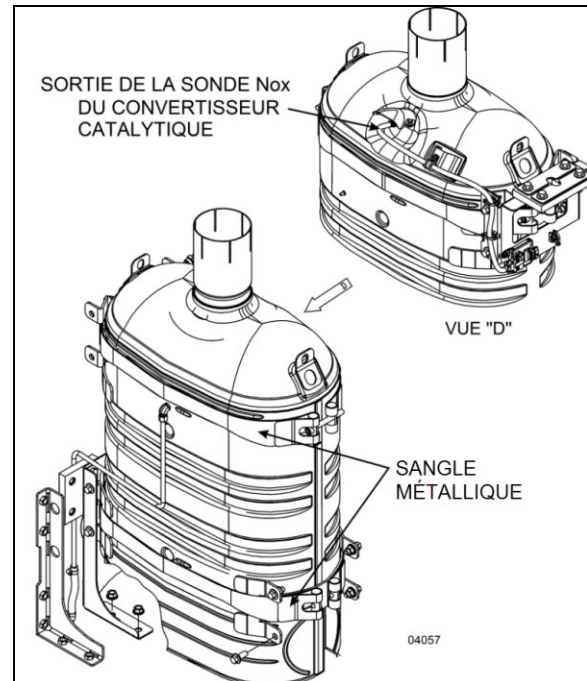
FIGURE 5: CONVERTISSEUR CATALYTIQUE
