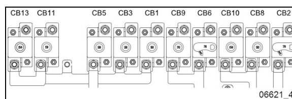
FIGURE 63 : PANNEAU DE JONCTION ÉLECTRIQUE ARRIÈRE SÉRIE X3, AVEC DISJONCTEURS
