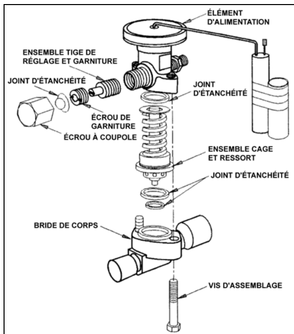
FIGURE 54 : DÉTENDEUR
