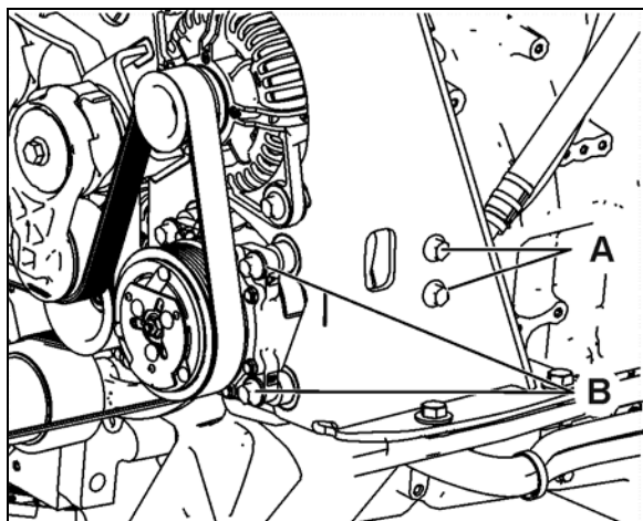
FIGURE 36: MONTAGE DU COMPRESSEUR DE LA SÉRIE X
