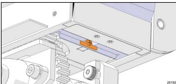
FIGURE 21: VIS DE FIXATION DU RIDEAU PROTECTEUR
