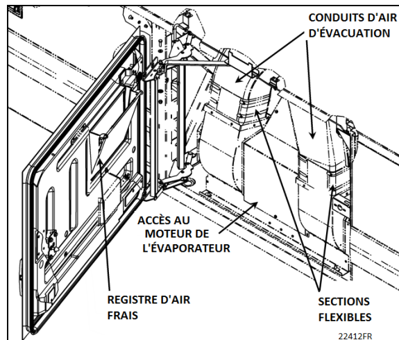
FIGURE 38: COMPARTIMENT DE L'ÉVAPORATEUR SÉRIE X3
