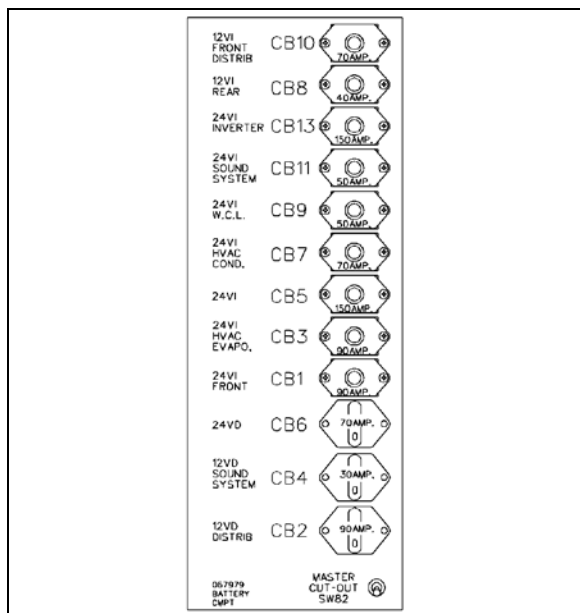
FIGURE 64: DISJONCTEURS DU CIRCUIT PRINCIPAL DES SÉRIES H3 6582A
