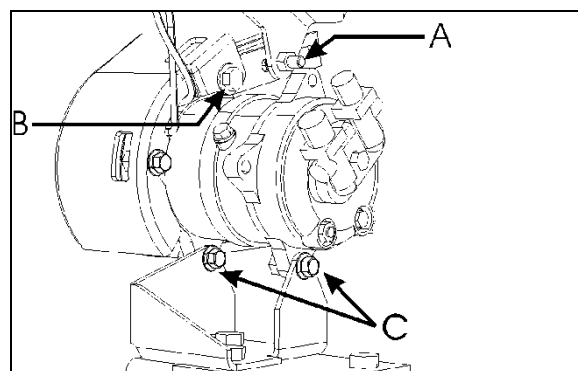
FIGURE 35: MONTAGE DU COMPRESSEUR DE LA SÉRIE H
