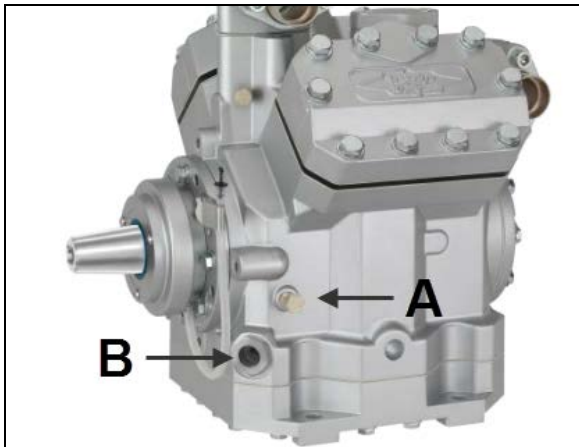
FIGURE 33: ORIFICE DE REMPLISSAGE (A) ET VERRE DE REGARD (B)
