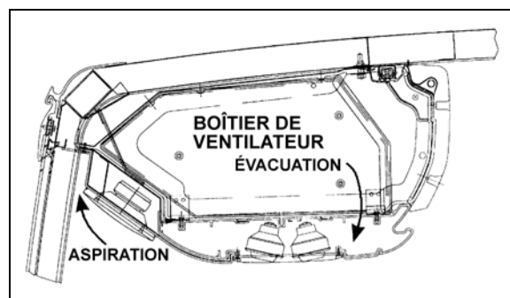
FIGURE 67 : SYSTÈME DE VENTILATION DU PORTE-BAGAGES À MAIN
