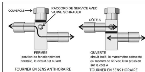
FIGURE 49 : ROBINET D'ARRÊT DU CIRCUIT DE REFROIDISSEMENT
