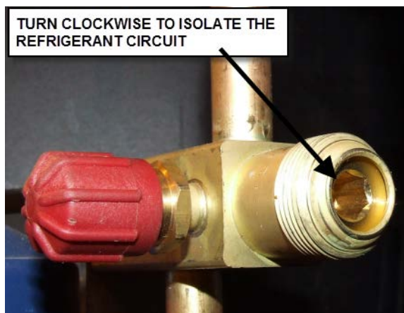
FIGURE 50 : ROBINET D'ARRÊT DU CIRCUIT DE REFROIDISSEMENT
