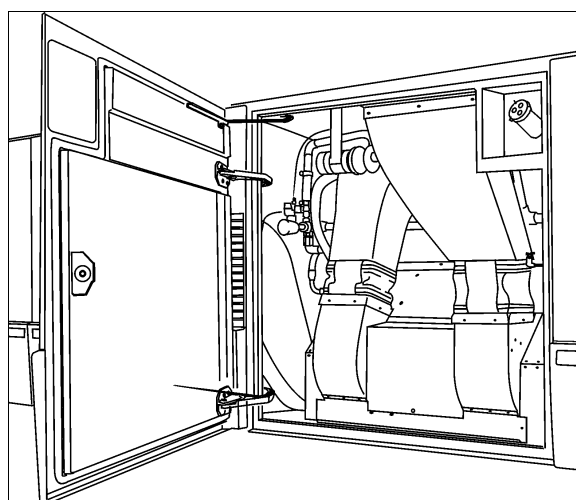
COMPARTIMENT DE L'ÉVAPORATEUR 22365
