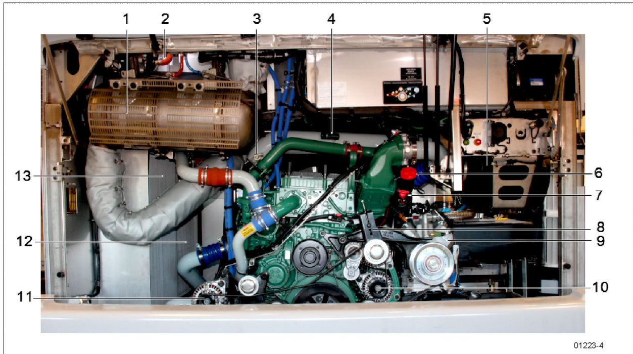
COMPARTIMENT MOTEUR ÉQUIPÉ DU MOTEUR VOLVO D13
