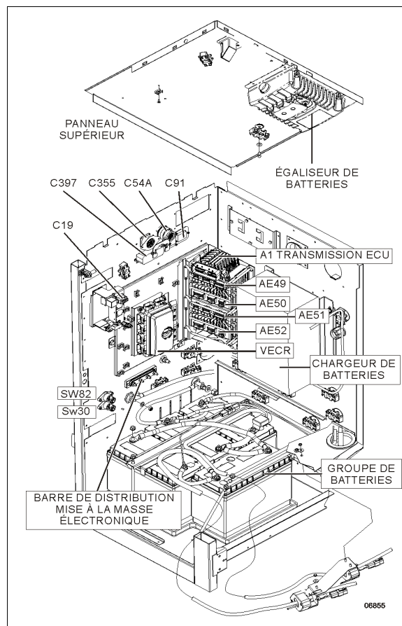
VUE PARTIELLE DU COMPARTIMENT PRINCIPAL D'ALIMENTATION
