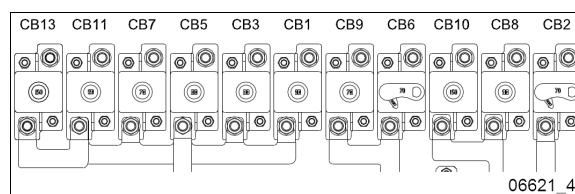
INTERRUPTEURS PRINCIPAUX 12 & 24 VOLTS
