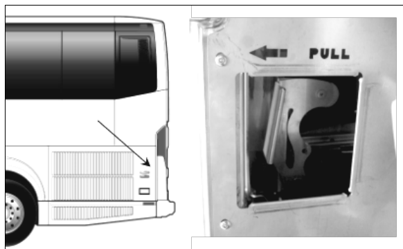
POSITION DU LOQUET PORTE DU RADIATEUR 18529_2
