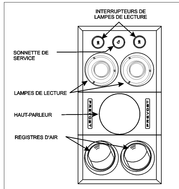
CONSOLE DE PASSAGER 23137
