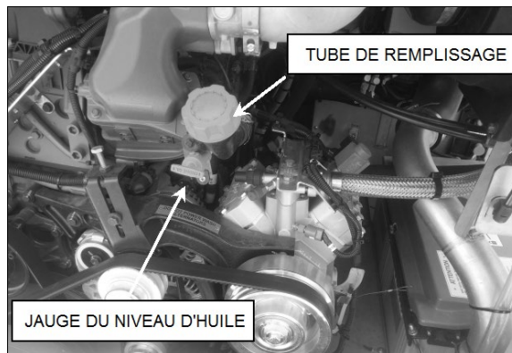
JAUGE ET TUBE DE REMPLISSAGE DU MOTEUR 01192_3
