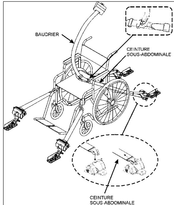
IMMOBILISATION DU FAUTEUIL ET FIXATION DE LA CEINTURE DE SÉCURITÉ
