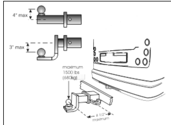
DISPOSITIF D'ATTELAGE
