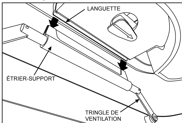
POIGNÉE D'OUVERTURE 23150
