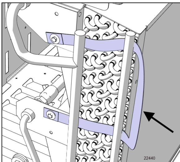
COURROIE
