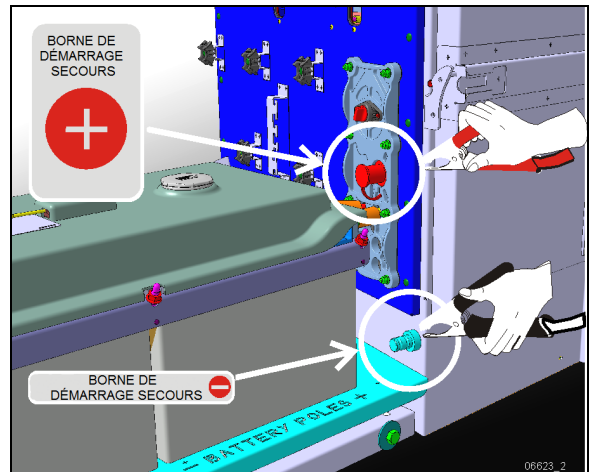
POSITION DES BORNES POUR DÉMARRAGE-SECOURS
