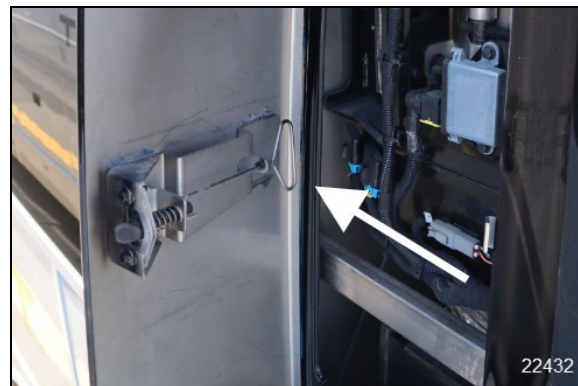
POIGNÉE D'OUVERTURE DE LA PORTE D'ACCÈS AU CONVERTISSEUR CATALYTIQUE
