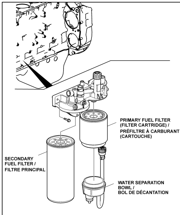
FILTRES À CARBURANT - MOTEUR VOLVO D13 03085
