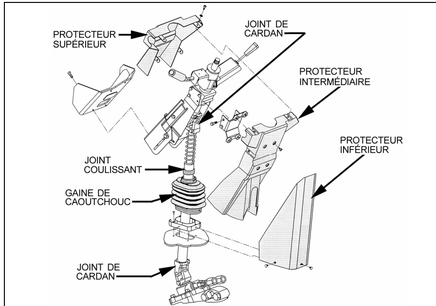
FIGURE 1: PROTECTEURS DE COLONNE DE DIRECTION
